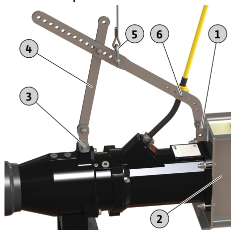
Fig. 21: Changer le châssis
