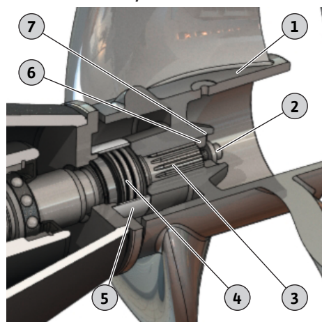
Fig. 15: Remplacement d'hélice OPTI-TR/EXCEL-TRE 50-3 à 80-3
