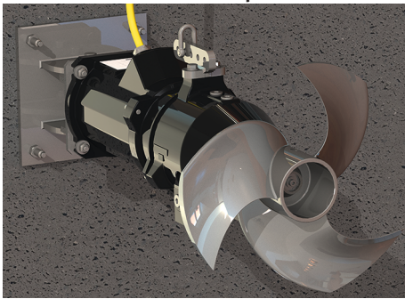
Fig. 3: Agitateur avec console sur la paroi du bassin
