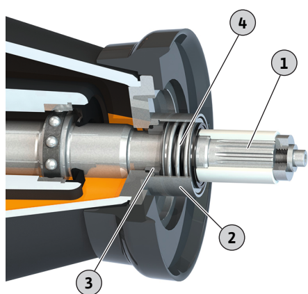
Fig. 20: Remplacer la garniture mécanique
