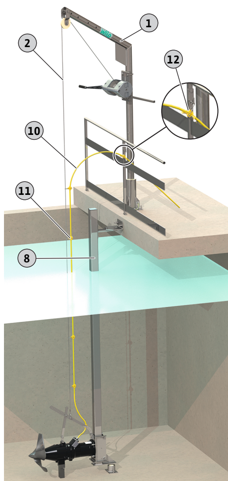
Fig. 10: Agitateur déposé sur la butée fixe
