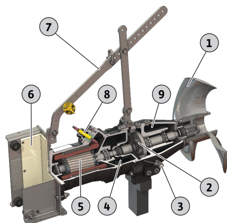
Fig. 2: Aperçu de l'agitateur submersible
