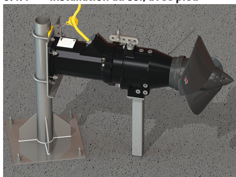
Fig. 5: Installation au sol, pied avec tuyau rond
