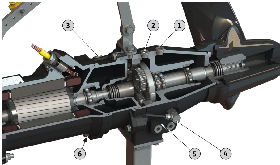
Fig. 13: Position des bouchons filetés
