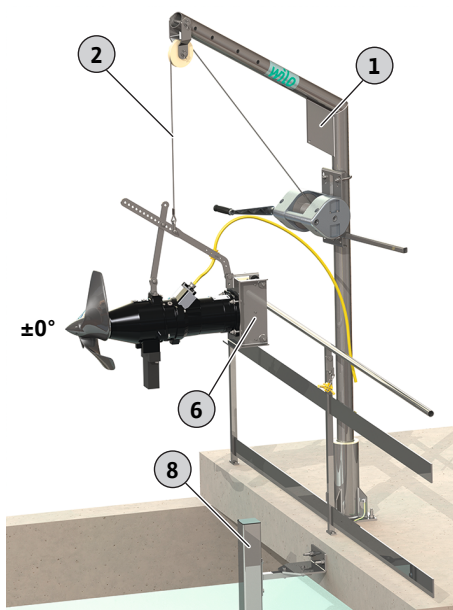
Fig. 8: Basculer l'agitateur au-dessus du bassin
