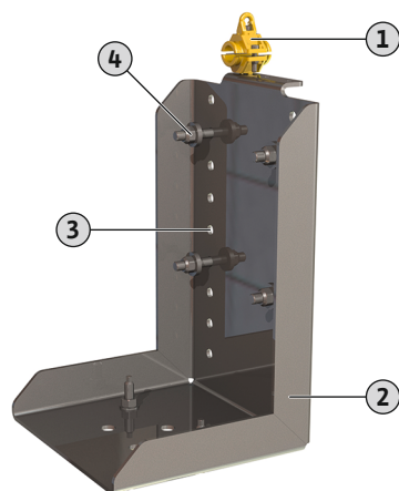
Fig. 23: Console pour montage au sol
