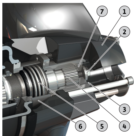
Fig. 19: Remplacement d'hélice OPTI-TR 120-1
