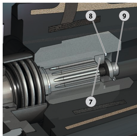
Fig. 17: Fixation de l'hélice
