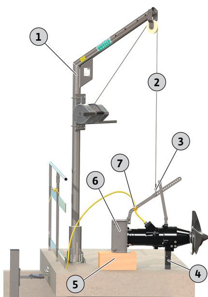
Fig. 7: Préparation de l'agitateur
