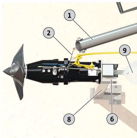
Fig. 9: Agitateur sur le dispositif de descente et support
