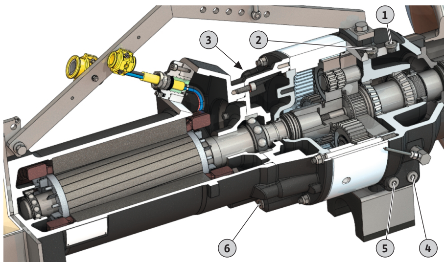
Fig. 14: Position des bouchons filetés
