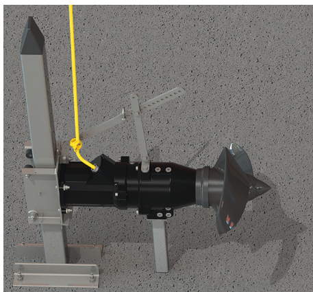
Fig. 6: Installation au sol, pied avec tuyau carré
