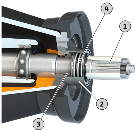
Fig. 20: Cambio de cierre mecánico
