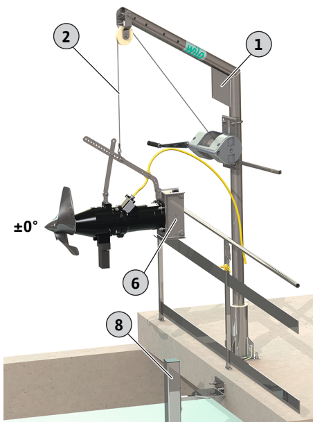
Fig. 8: Giro del agitador sobre el depósito
