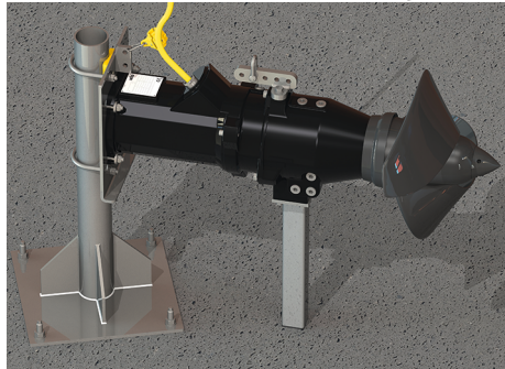
Fig. 5: Instalación en la base, pedestal con tubo redondo
