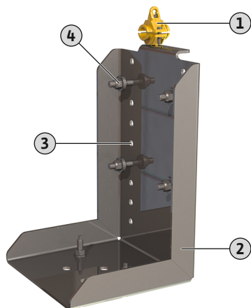
Fig. 23: Soporte para el montaje sobre el suelo
