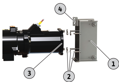
Fig. 22: Sustitución del bastidor
