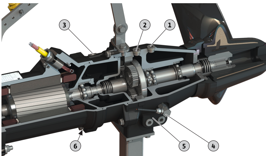
Fig. 13: Posición de los tapones roscados
