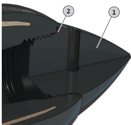
Fig. 18: Tapa del buje con junta tórica
