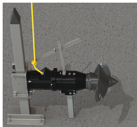
Fig. 6: Instalación en la base, pedestal con tubo cuadrado
