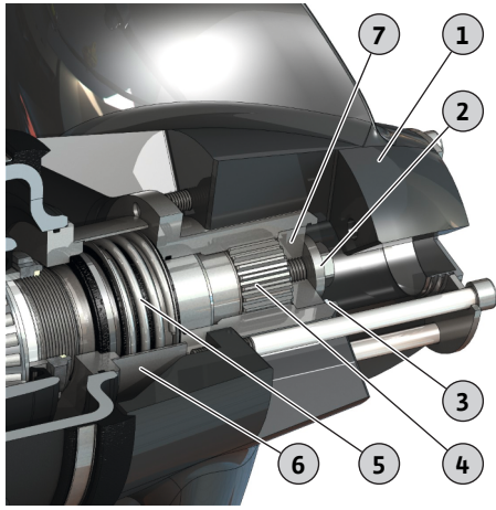
Fig. 19: Cambio de hélice OPTI-TR 120-1
