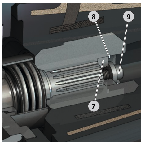
Fig. 17: Fijación de la hélice
