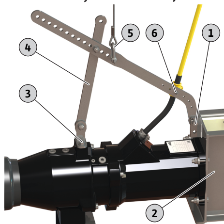
Fig. 21: Sustitución del bastidor
