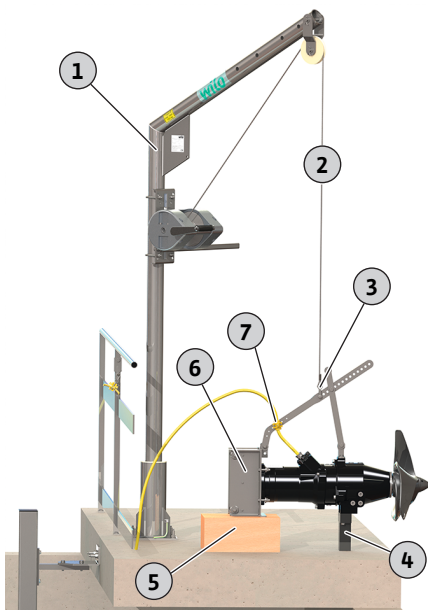
Fig. 7: Preparar el agitador
