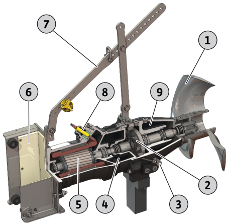
Fig. 2: Vista general del agitador de motor sumergible
