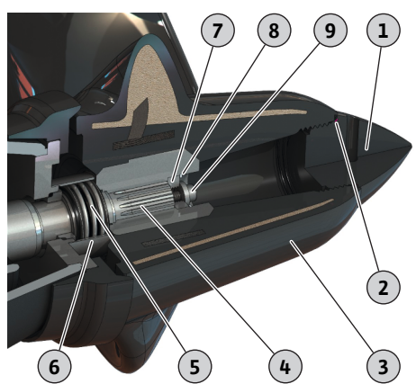
Fig. 16: Αντικατάσταση έλικα OPTI-TR/EXCEL-TRE 90-2
