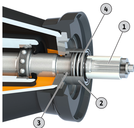
Fig. 20: Αντικατάσταση μηχανικού στυπιοθλίπτη
