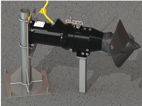
Fig. 5: Εγκατάσταση στον πυθμένα, ορθοστάτης με στρογγυλό σωλήνα
