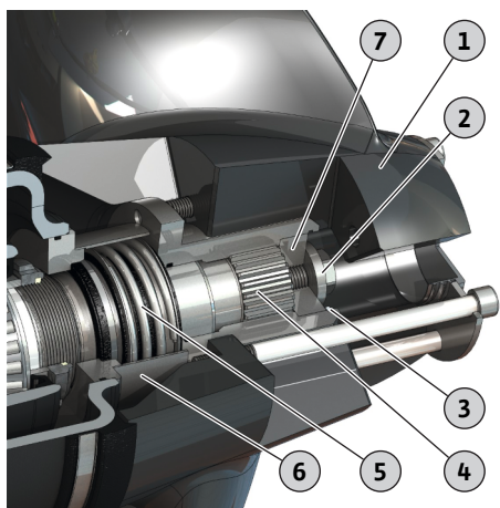
Fig. 19: Αντικατάσταση έλικα OPTI-TR 120-1
