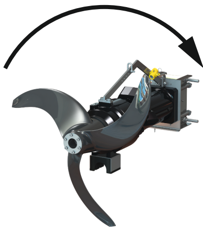
Fig. 12: Σωστή φορά περιστροφής
