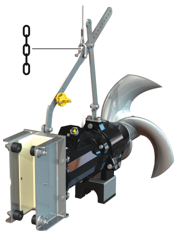
Fig. 1: Σημείο πρόσδεσης
