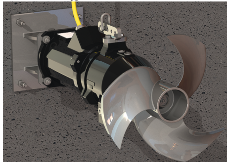
Fig. 3: Αναδευτήρας με υποστήριγμα στερέωσης στο τοίχωμα της λεκάνης
