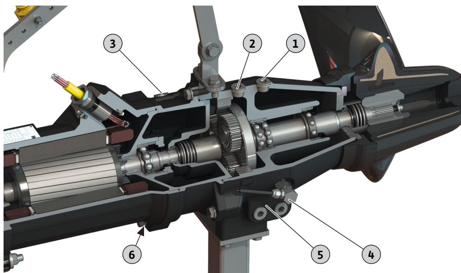
Fig. 13: Θέση των βιδωτών ταπών
