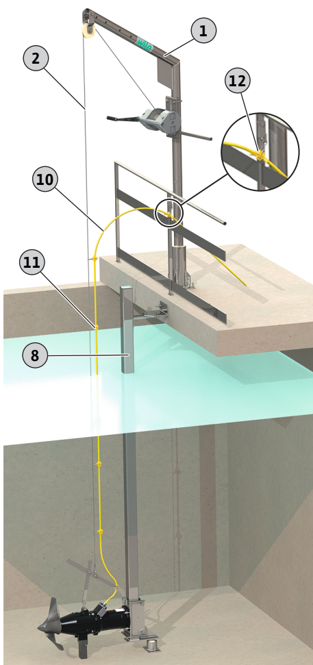
Fig. 10: Αναδευτήρας τοποθετημένος σε σταθερό τερματικό σημείο
