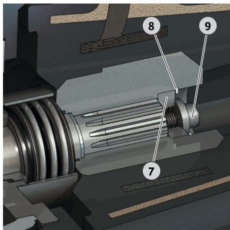
Fig. 17: Στερέωση έλικα
