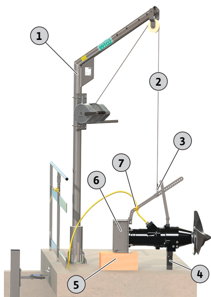
Fig. 7: Προετοιμασία αναδευτήρα
