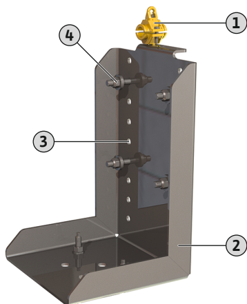
Fig. 23: Υποστήριγμα στερέωσης για επιδιπέδια εγκατάσταση
