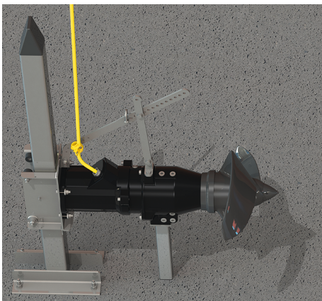
Fig. 6: Εγκατάσταση στον πυθμένα, ορθοστάτης με τετραγωνικό σωλήνα
