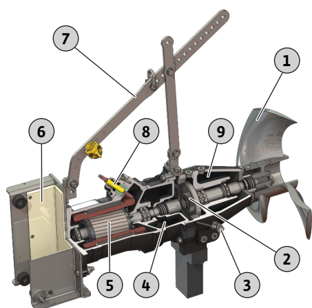
Fig. 2: Επισκόπηση υποβρύχιου αναδευτήρα
