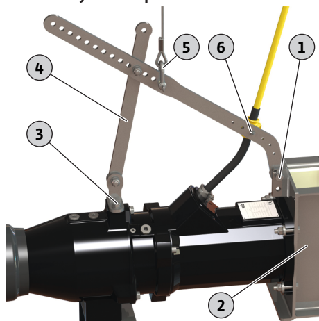
Fig. 21: Výmena rámu
