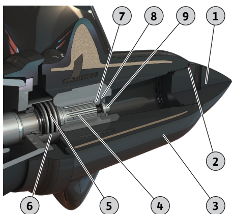
Fig. 16: Výmena vrtule OPTI-TR/EXCEL-TRE 90-2
