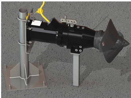
Fig. 5: Inštalácia na dno so statívom s okrúhrou rúrou
