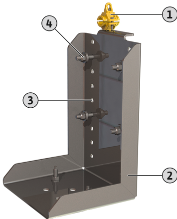
Fig. 23: Konzola pre montáž na dno
