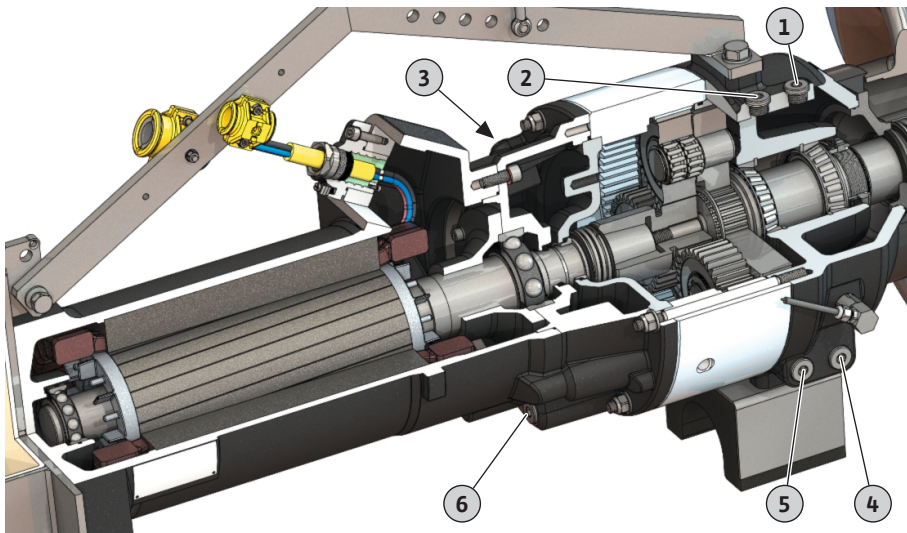
Fig. 14: Umiestnenie uzatváracích skrutiek
