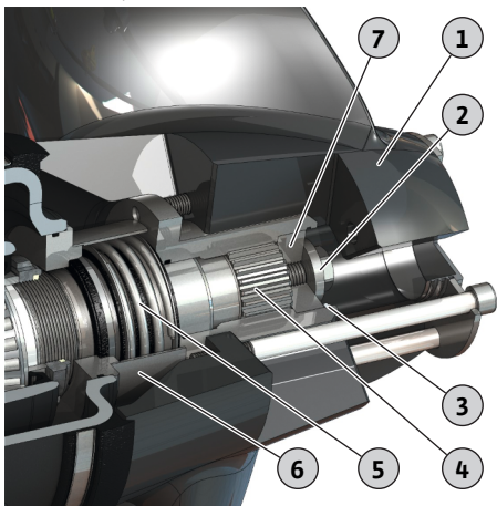
Fig. 19: Výmena vrtule OPTI-TR 120-1
