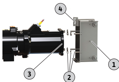
Fig. 22: Výmena rámu
