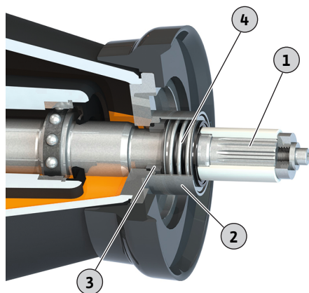
Fig. 20: Výmena mechanickej upchávky
