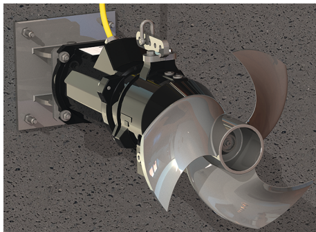
Fig. 3: Miešacie zariadenie s konzolou na stenu nádrže
