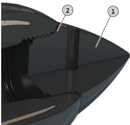
Fig. 18: Uzatvárací kryt náboja s O-krúžkom
