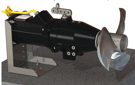
Fig. 4: Miešacie zariadenie s konzolou na dno nádrže
