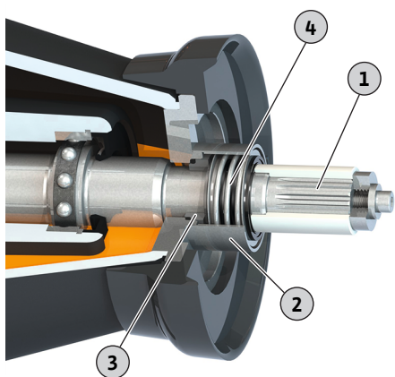
Fig. 20: Byte av mekanisk tätning
