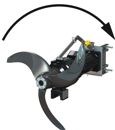
Fig. 12: Rätt rotationsriktning
