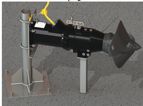
Fig. 5: Installation på golvet, stativ med rundrör
