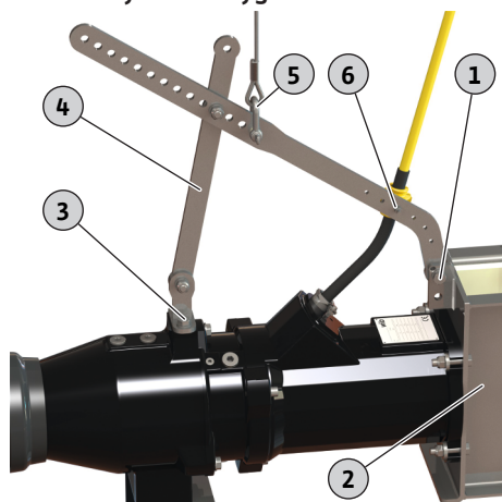
Fig. 21: Byte av ramen
