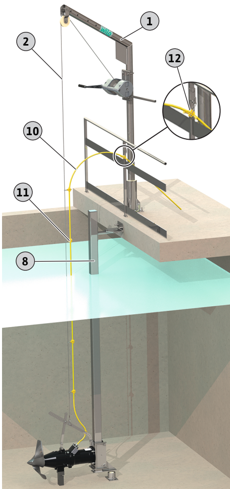
Fig. 10: Omrörare nedsänkt till fast stopp
