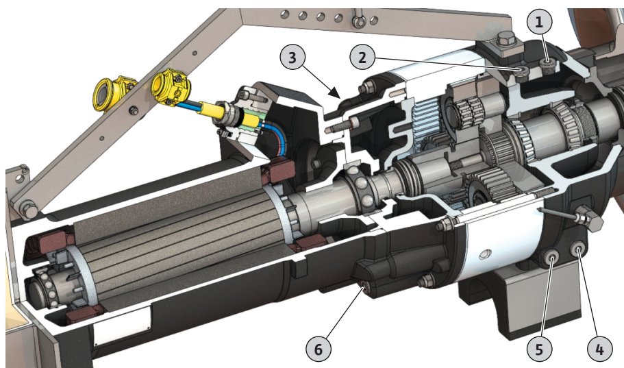
Fig. 14: Skruvpluggarnas placering
