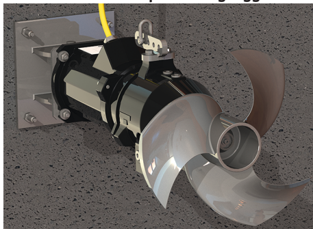
Fig. 3: Omrörare med konsol på bassängväggen
