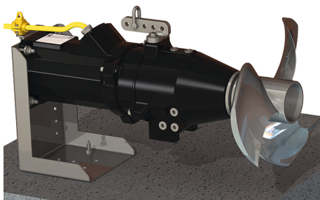
Fig. 4: Omrörare med konsol på bassänggolvet
