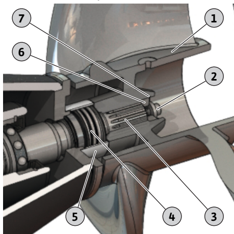
Fig. 15: Propellerbyte OPTI-TR/EXCEL-TRE 50-3 till 80-3
