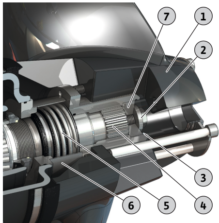
Fig. 19: Propellerbyte OPTI-TR 120-1
