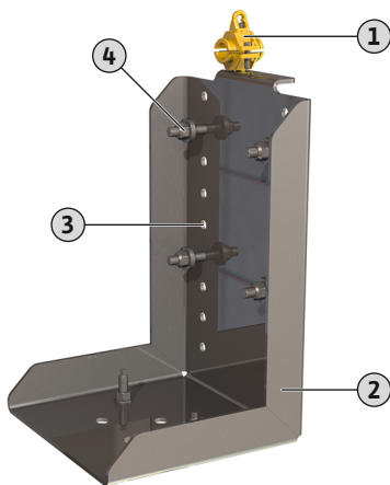
Fig. 23: Konsol för golvmontage
