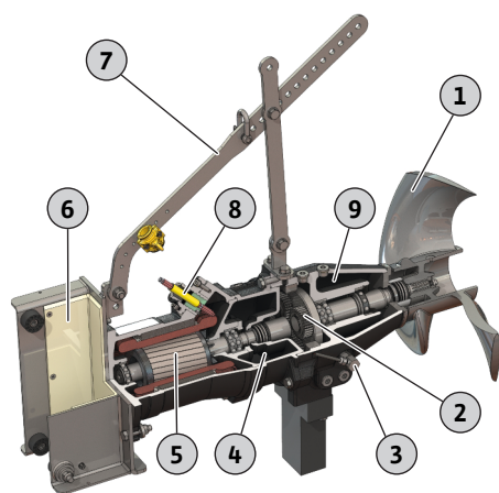
Fig. 2: Översikt över dränkbar omrörare
