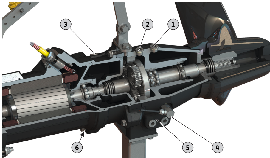
Fig. 13: Posição dos parafusos de fecho
