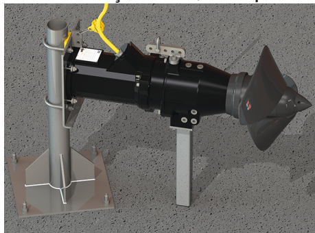
Fig. 5: Instalação no chão, tripé com tubo redondo
