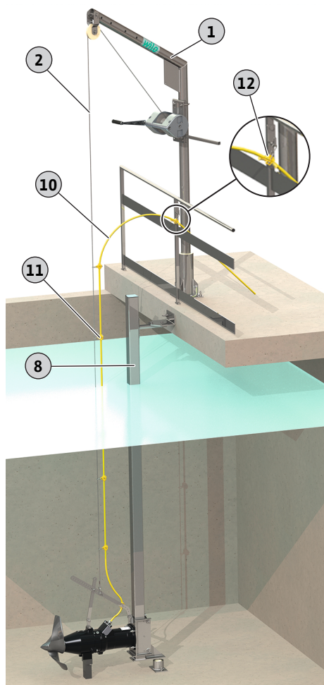
Fig. 10: Colocar o mecanismo agitador sobre o limite de parada fixado
