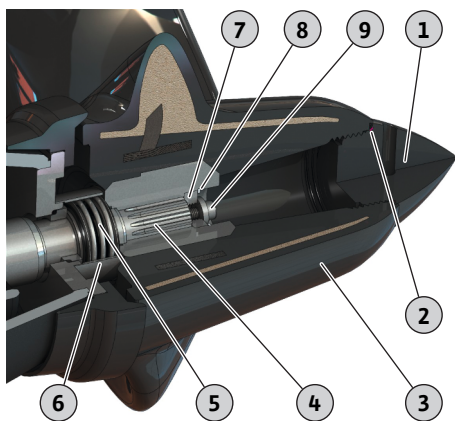
Fig. 16: Substituição da hélice OPTI-TR/ EXCEL-TRE 90-2
