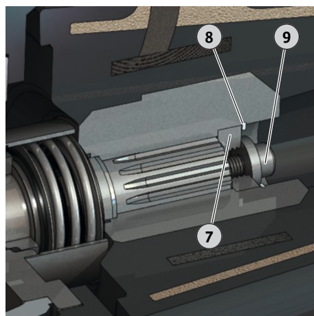
Fig. 17: Fixação da hélice
