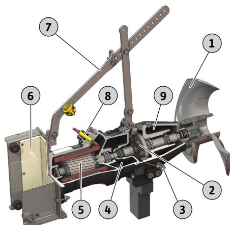
Fig. 2: Vista geral do mecanismo agitador de motor submersível
