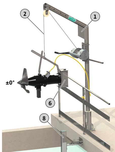
Fig. 8: Oscilar o mecanismo agitador sobre o tanque
