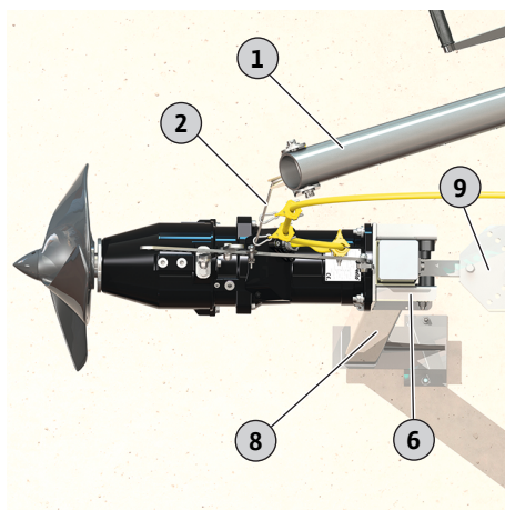
Fig. 9: Mecanismo agitador no dispositivo de abaixamento
