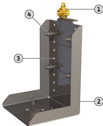
Fig. 23: Consola para montagem no solo
