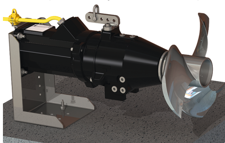
Fig. 4: Mecanismo agitador com consola no fundo do tanque
