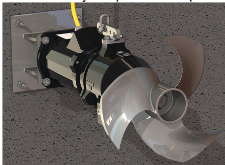
Fig. 3: Mecanismo agitador com consola na parede do tanque
