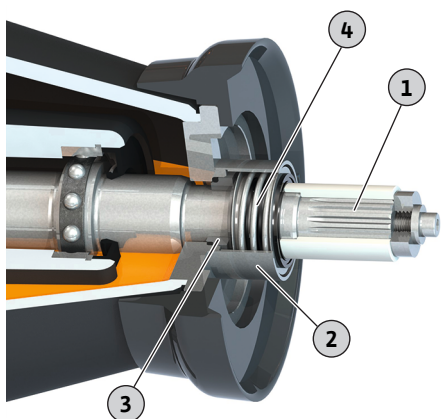
Fig. 20: Substituição do empanque mecânico
