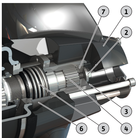
Fig. 19: Substituição da hélice OPTI-TR 120-1
