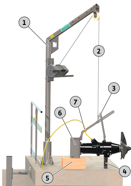
Fig. 7: Preparar o mecanismo agitador
