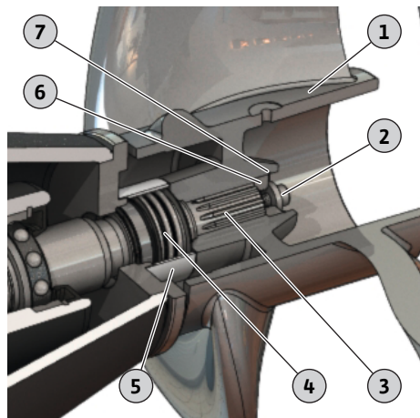
Fig. 15: Substituição da hélice OPTI-TR/EXCEL-TRE 50-3 até 80-3
