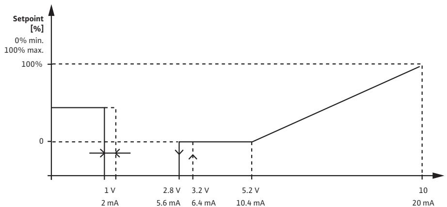
Fig. 34: Sollwerteingang 2 – 10 V bzw. 4 – 20 mA
