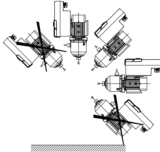
Fig. 5: Zulässige Einbaulagen mit Motorwelle und Elektronikmodul nach oben (0°)
