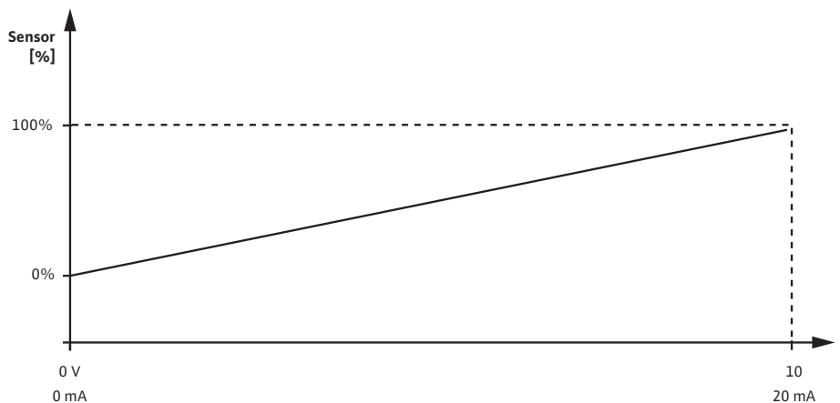
Fig. 35: Sensoreingang 0 – 10 V oder 0 – 20 mA
