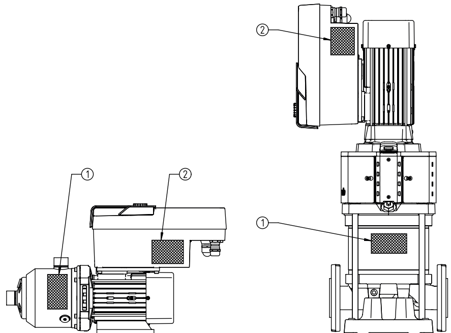
Fig. 3: Typenschilder
