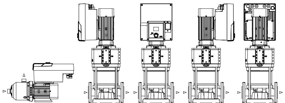
Fig. 4: Anordnung der Komponenten im Lieferzustand
