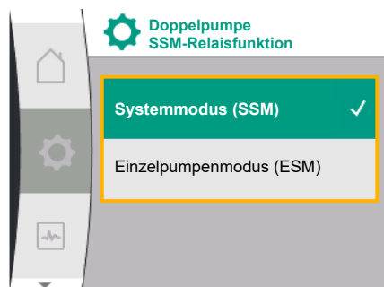
Fig. 28: Menü Doppelpumpe SSM-Relaisfunktion
