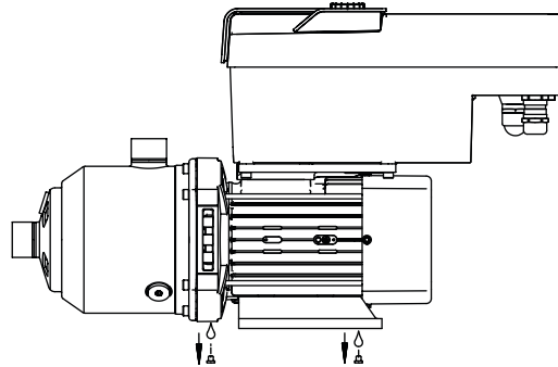
Fig. 6: Kondensatablauföffnungen
