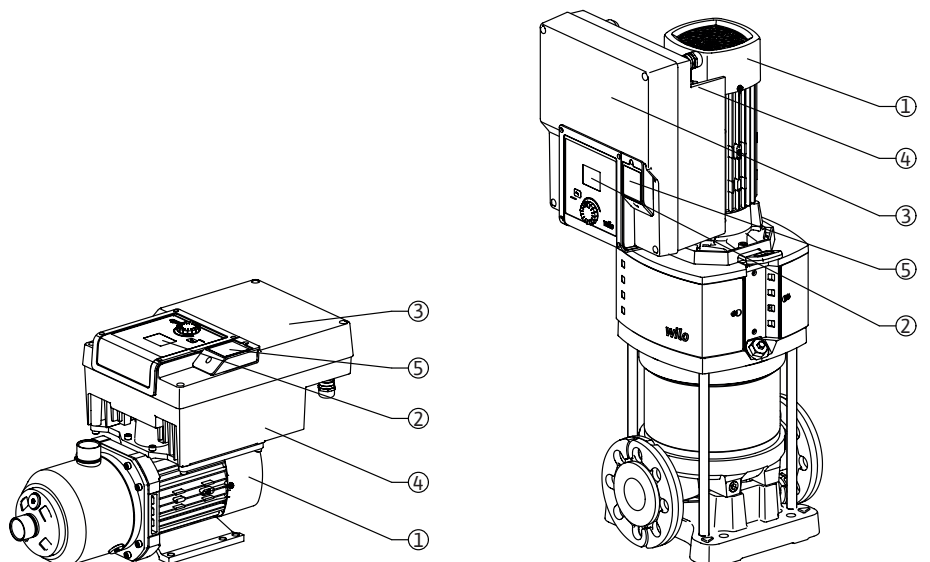
Fig. 2: Antriebsübersicht
