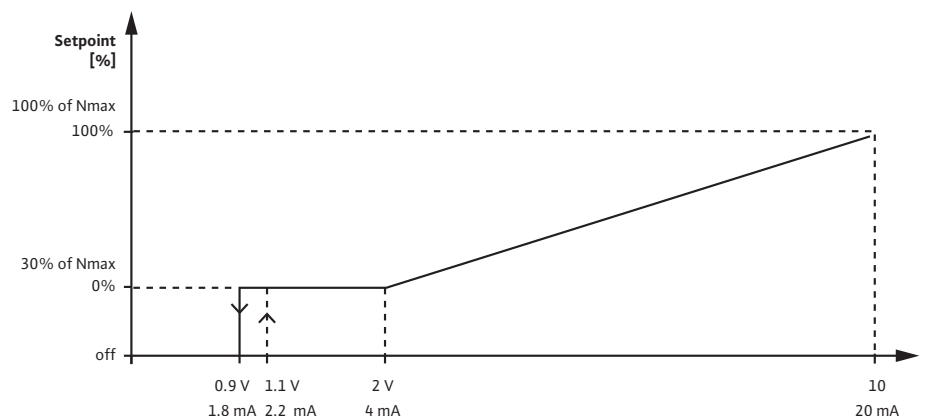
Fig. 33: Sollwerteingang 0 – 10 V oder 0 – 20 mA
