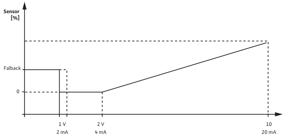
Fig. 36: Sensoreingang 0 – 10 V oder 0 – 20 mA
