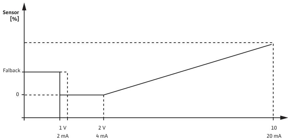
Fig. 36: Вхід давача 0 – 10 В або 0 – 20 мА
