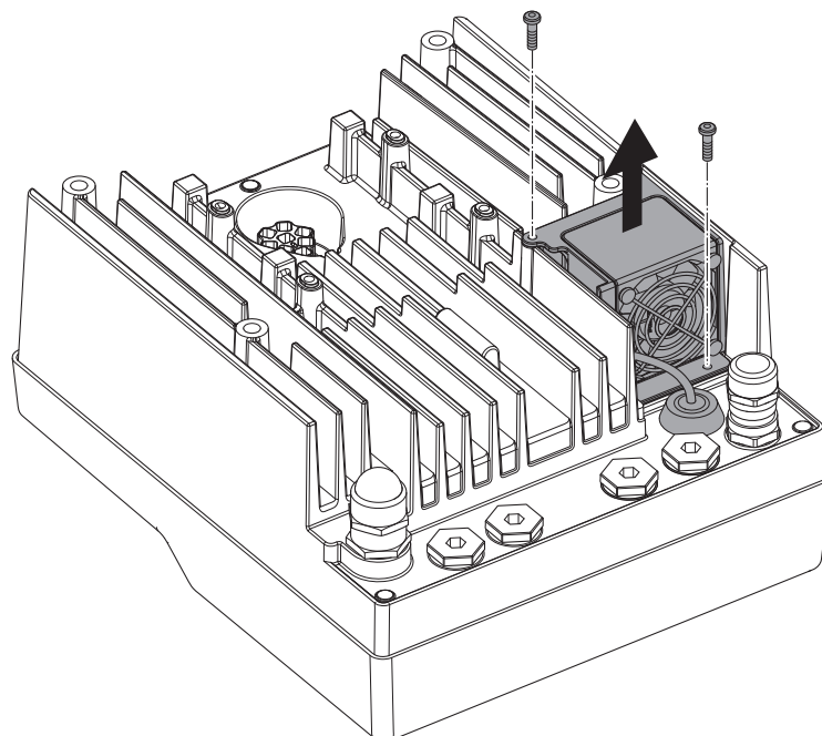
Fig. 44: Демонтаж вентилятора модуля
