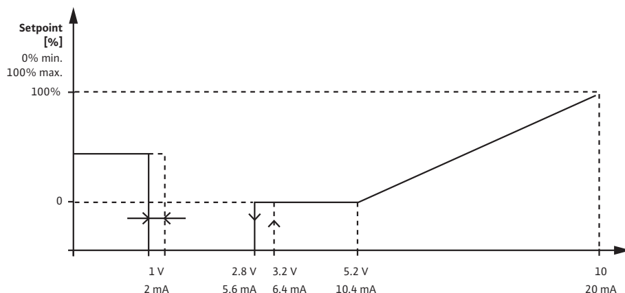
Fig. 34: Вхід заданого значення 2 – 10 В або 4 – 20 мА
