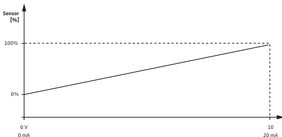
Fig. 35: Вхід давача 0 – 10 В або 0 – 20 мА
