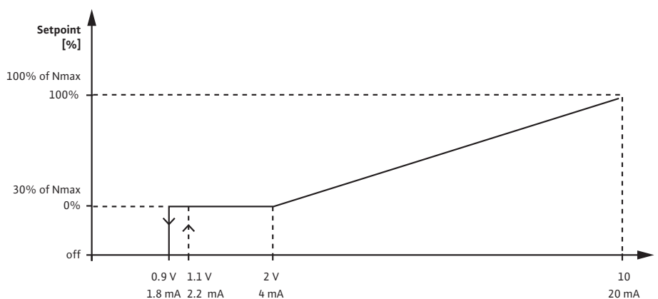
Fig. 33: Вхід заданого значення 0 – 10 В або 0 – 20 mA
