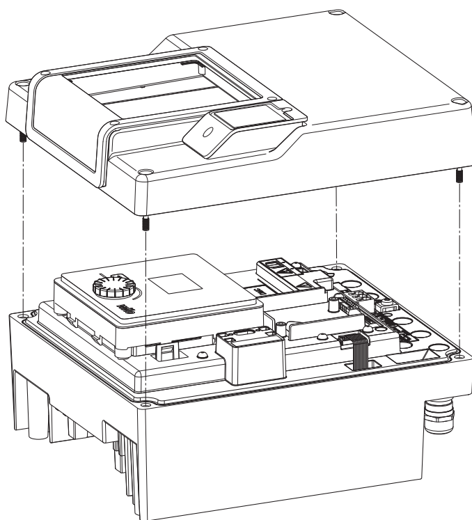
Fig. 42: Відкривання кришки електронного модуля
