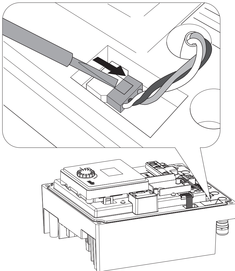
Fig. 43: Від'єднання під'єднувального кабелю вентилятора модуля
