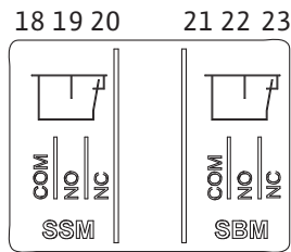
Fig. 15: Клеми для SSM і SBM
