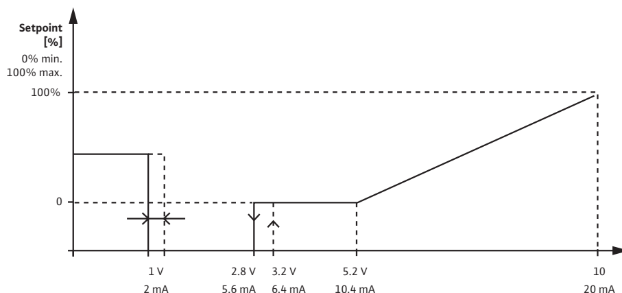
Fig. 34: Vhodna želena vrednost 2 – 10 V oz. 4 – 20 mA
