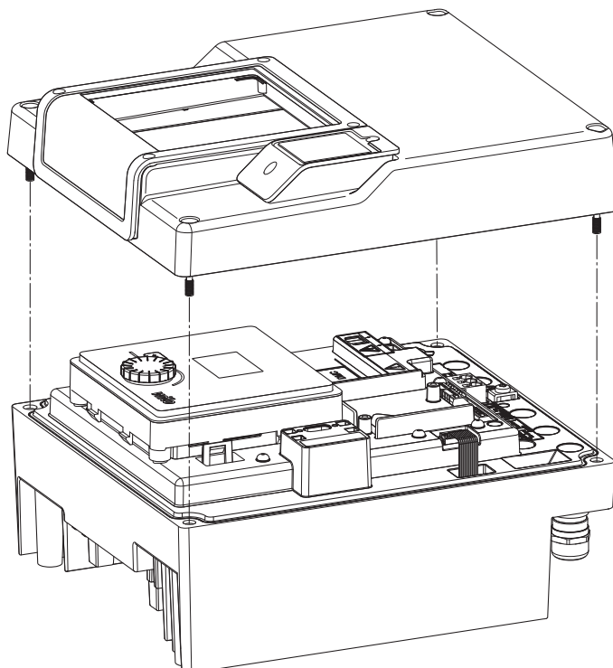
Fig. 42: Odpiranje pokrova elektronskega modula
