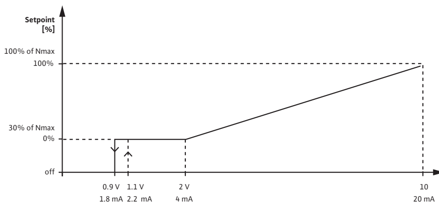
Fig. 33: Reikiamos darbinės vertės įeiga 0–10 V arba 0–20 mA
