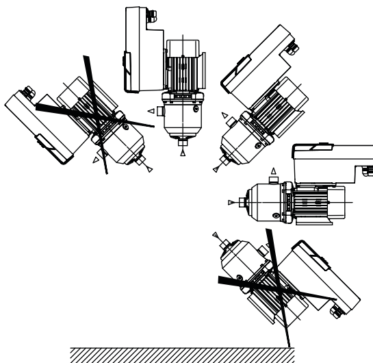
Fig. 5: Leistinos montavimo padėtys su variklio vėlenu ir į viršų nukreiptu elektronikos modulių (0°)
