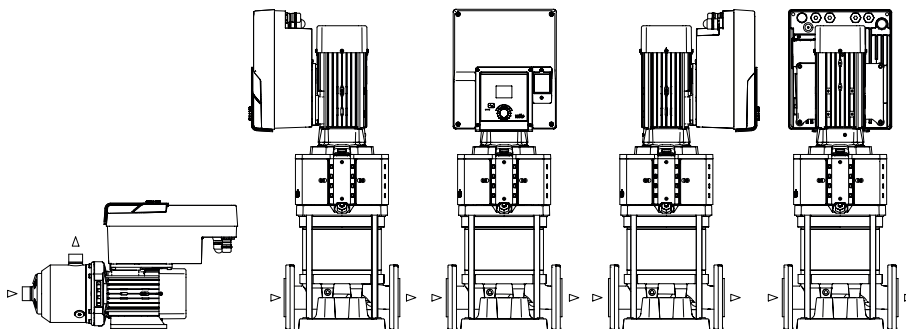
Fig. 4: Komponentų išdėstymo tvarka tiekimo komplektacijoje
