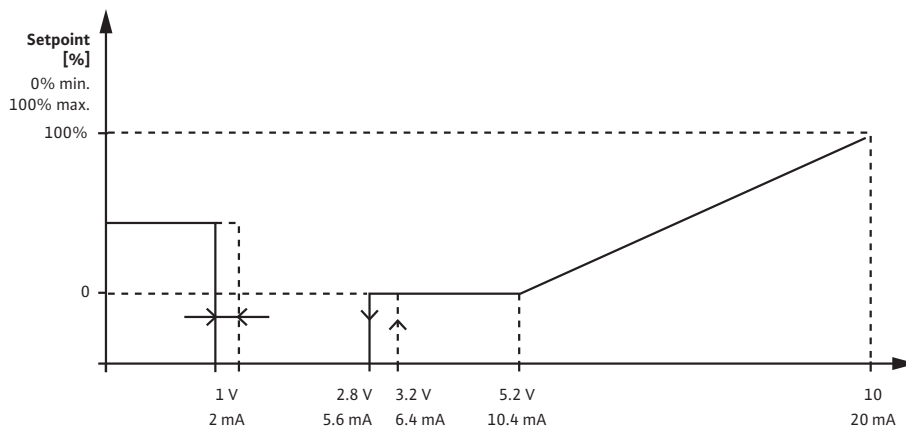
Fig. 34: Reikiamos darbinės vertės įeiga 2–10 V arba 4–20 mA
