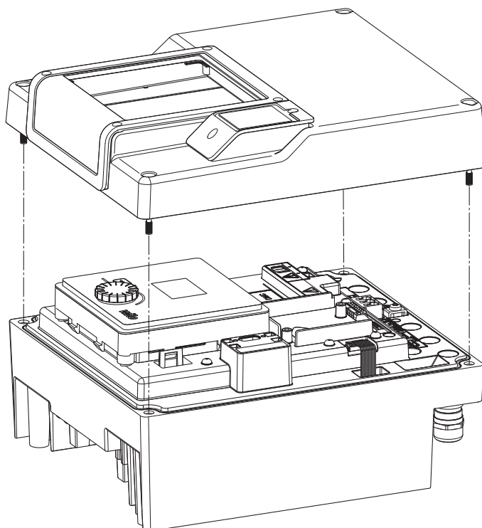
Fig. 42: Elektroniikkamoduulin kannen avaaminen
