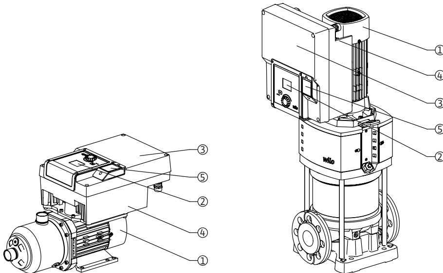
Fig. 2: Käyttömoottorin yleiskatsaus
