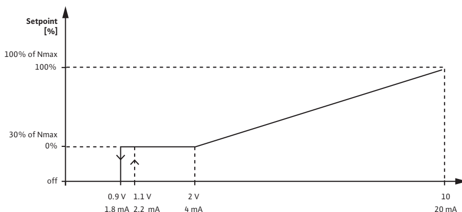
Fig. 33: Asetusarvon tulo 0–10 V tai 0–20 mA
