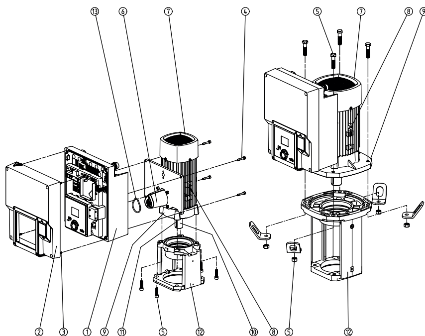
Fig. 1: Tärkeimmät osat
