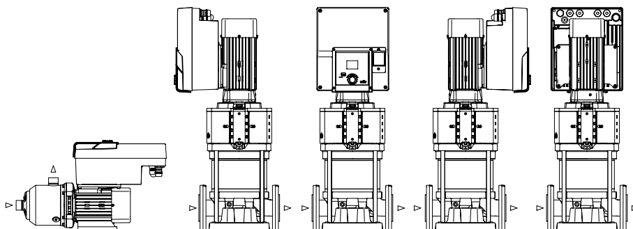
Fig. 4: Komponenttien sijainti toimitustilassa
