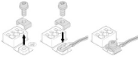
Fig. 14: Jäykkä liitäntäkaapeli
