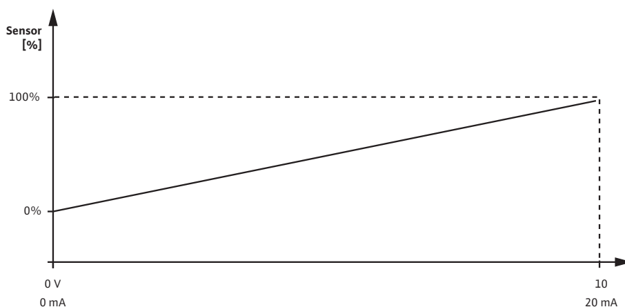
Fig. 35: Anturitulo 0–10 V tai 0–20 mA
