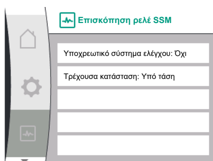
Fig. 39: Επισκόπηση της λειτουργίας ρελέ SSM
