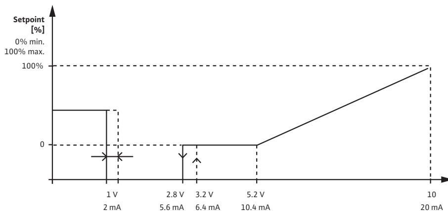
Fig. 34: Είσοδος επιθυμητής τιμής 2 – 10 V ή 4 – 20 mA
