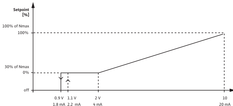
Fig. 33: Είσοδος επιθυμητής τιμής 0 – 10 V ή 0 – 20 mA
