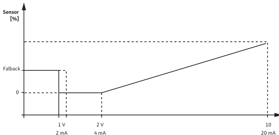
Fig. 36: Είσοδος αισθητήρα 0 – 10 V ή 0 – 20 mA
