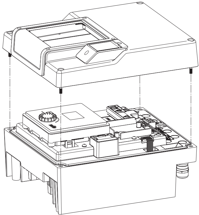
Fig. 42: Ανοίξτε το κάλυμμα της ηλεκτρονικής μονάδας
