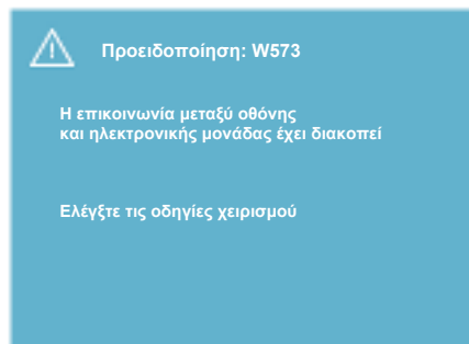
Fig. 41: Προειδοποίηση
