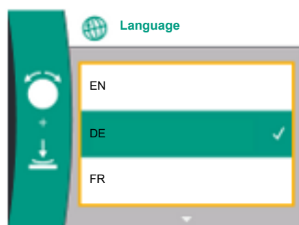
Fig. 23: Μενού ρυθμίσεων
