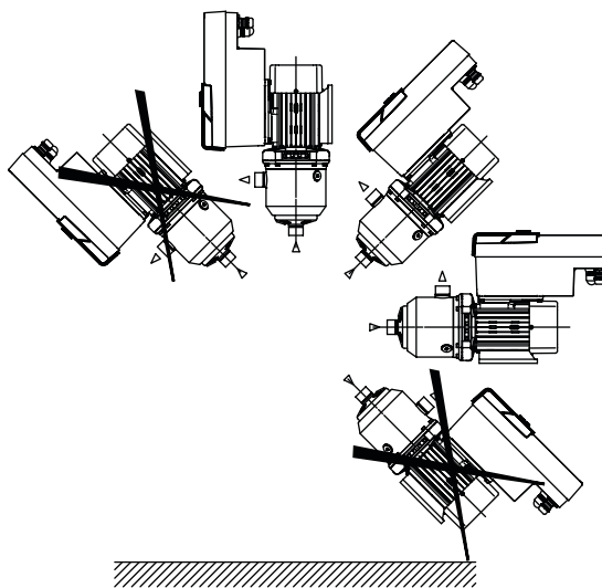
Fig. 5: Οι επιτρεπόμενες θέσεις τοποθέτησης με άξονα κινητήρα και με ηλεκτρονική μονάδα προς τα πάνω (0°)
