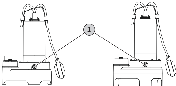
Fig. 6: Výměna oleje těsnicí komory
