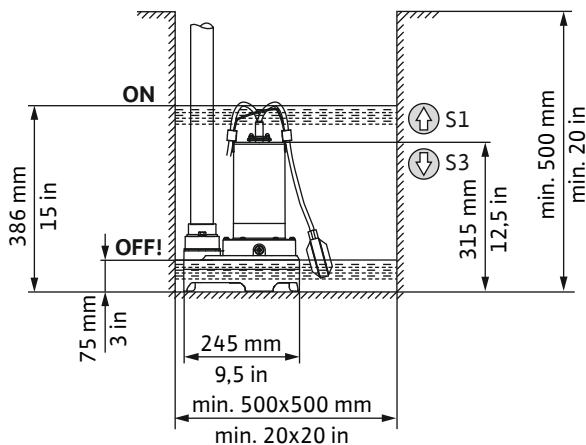
Fig. 2: Padus MINI3-M: Rozměry pro instalaci a spínací body
