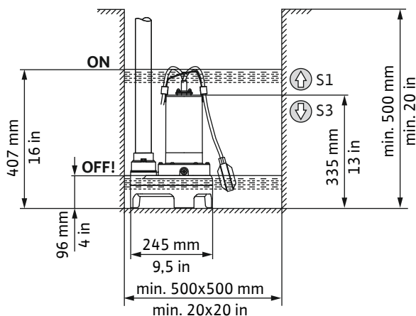
Fig. 3: Padus MINI3-V: Rozměry pro instalaci a spínací body
