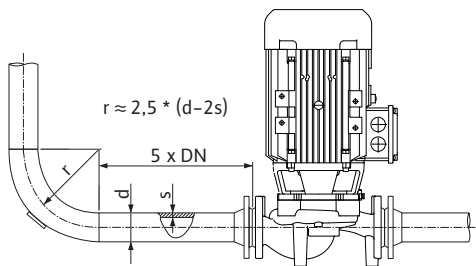
Fig. 9: Deonica za stabilizaciju ispred i iza pumpe
