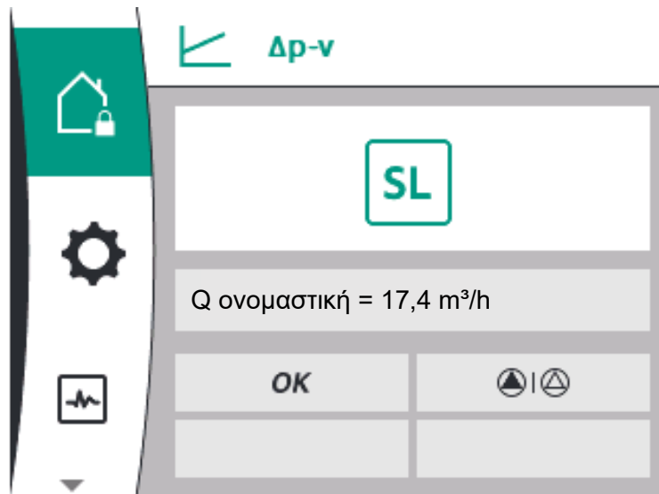
Fig. 59: Αρχική οθόνη συνεργάτη διδυμων αντλιών
