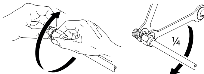
Fig. 13: Περιστρέψτε τη βιδωτή σύνδεση σύσφιγξης κατά 1/4
