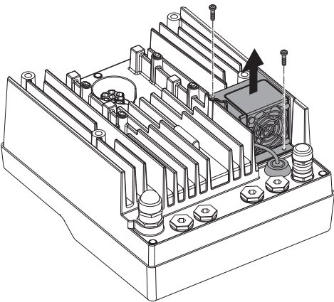
Fig. 104: Αποσυναρμολόγηση του ανεμιστήρα στοιχείου
