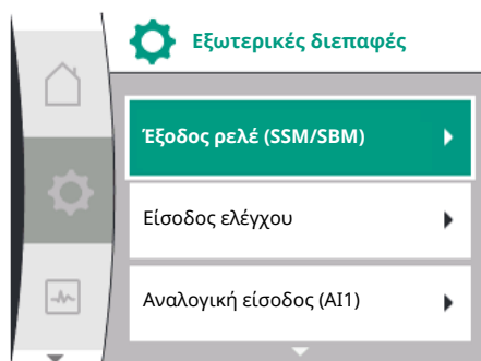
Fig. 60: Μενού εξωτερικές διεπαφές
