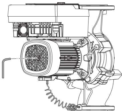
Fig. 5: Περιστροφή του άξονα
