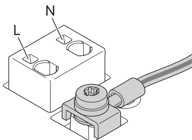
Fig. 23: Ακροδέκτης ηλεκτρικού δικτύου για ηλεκτρική σύνδεση 1~ με γείωση
