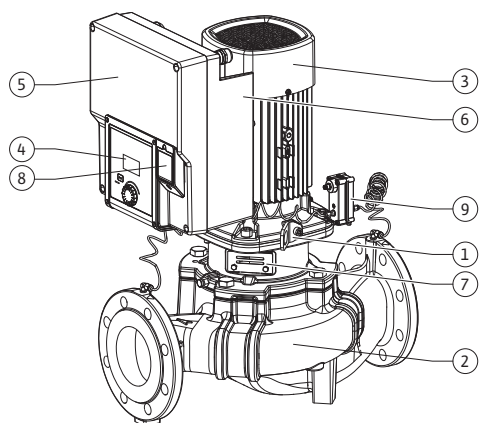
Fig. 1: Επισκόπηση αντλίας
