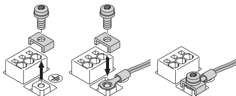
Fig. 24: Εύκαμπτο καλώδιο σύνδεσης
