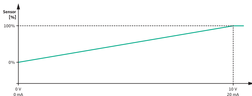
Fig. 73: Συμπεριφορά αναλογικής εισόδου AI1: Τιμή αισθητήρα σε τύπο σήματος 0 ... 10 V / 0 ... 20 mA
