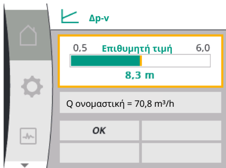
Fig. 34: Αρχική οθόνη – αλλαγή επιθυμητής τιμής Δp-v
