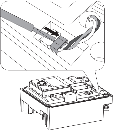
Fig. 103: Ξεσφίξτε το καλώδιο σύνδεσης του ανεμιστήρα στοιχείου
