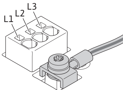
Fig. 22: Ακροδέκτης ηλεκτρικού δικτύου για ηλεκτρική σύνδεση 3~ με γείωση
