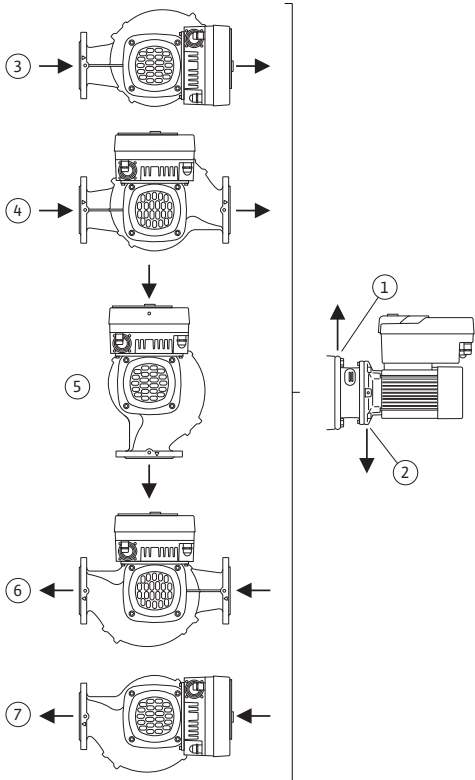
Fig. 9: Επιτρεπόμενες θέσεις τοποθέτησης με οριζόντιο άξονα κινητήρα
