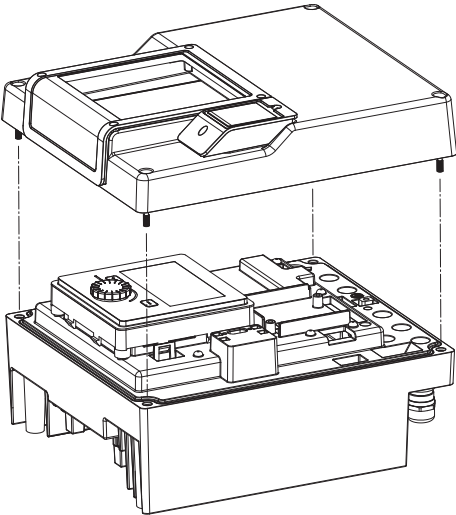
Fig. 102: Ανοίξτε το κάλυμμα της ηλεκτρονικής μονάδας
