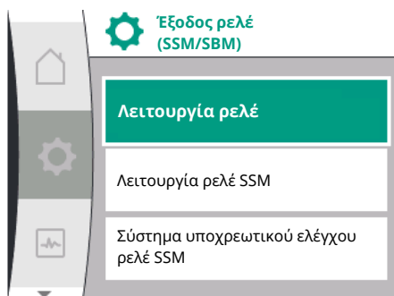
Fig. 61: Μενού εξόδου ρελέ SSM/SBM
