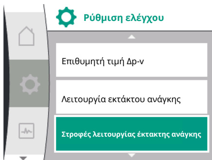
Fig. 71: Μενού ρυθμίσεων ελέγχου με λειτουργία έκτακτης ανάγκης σε περίπτωση βλάβης της τιμής του αισθητήρα
