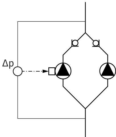
Fig. 18: Παράδειγμα - σύνδεση αισθητήρα διαφορικής πίεσης σε διχλωτές σωληνώσεις
