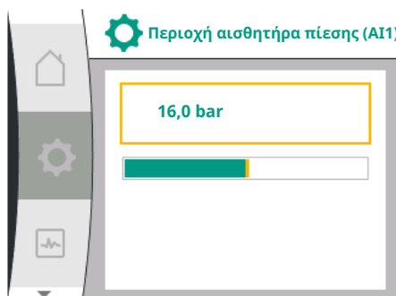
Fig. 69: Ρύθμιση εύρος αισθητήρα πίεσης
