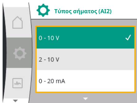
Fig. 75: Μενού τύπου σήματος (AI2)
