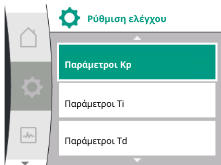
Fig. 43: Ρύθμιση παραμέτρων PID
