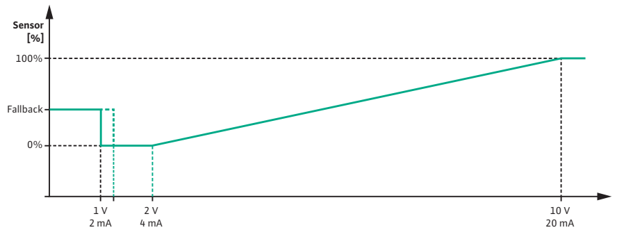
Fig. 70: Συμπεριφορά αναλογικής εισόδου AI 1: Τιμή αισθητήρα σε τύπο σήματος 2 ... 10 V / 4 ... 20 mA
