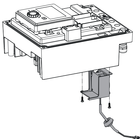
Fig. 105: Αφαιρέστε τον ανεμιστήρα στοιχείου μαζί με το καλώδιο και την ελαστική στεγανοποίηση
