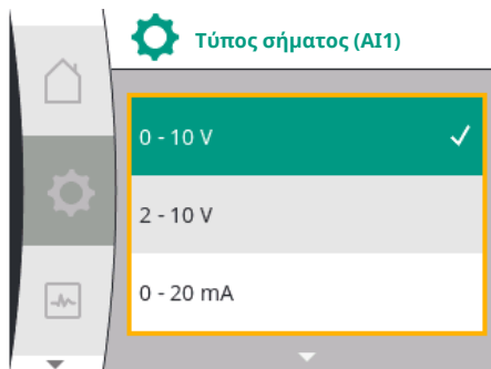
Fig. 68: Μενού τύποι σήματος
