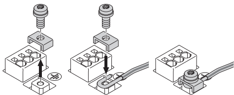
Fig. 25: Άκαμπτο καλώδιο σύνδεσης
