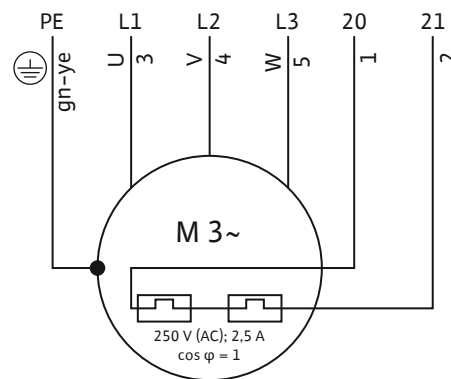
Fig. 5: Схемата на свързване 3~ мотор
