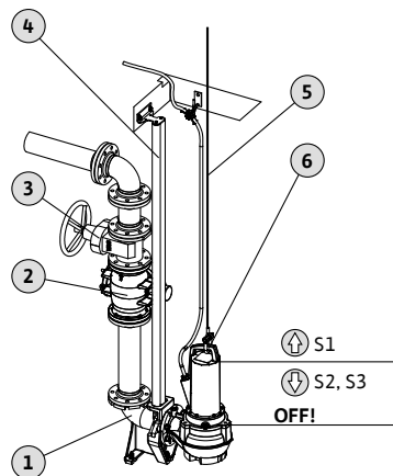
Fig. 4: Märkäasennus, kiinteä
