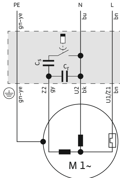
Fig. 6: Liitäntäkaavio 1~-moottori
