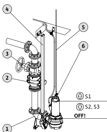
Fig. 4: Märkäasennus, kiinteä
