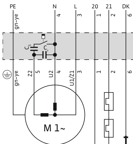
Fig. 6: Liitانتäkaavio 1~moottori
