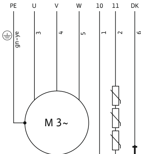
Fig. 8: Liitäntäkaavio 3~moottori: Suorakäynnistys, PTC-anturi
