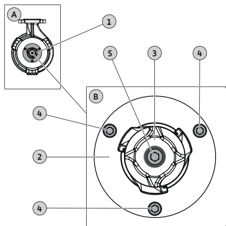
Fig. 10: Silppurin vaihto
