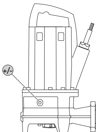
Fig. 9: Tiivistekammio: Öljyn vaihto
