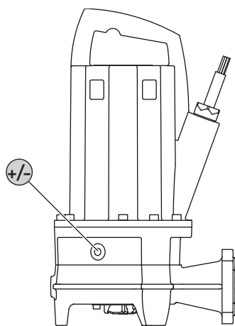
Fig. 9: Chambre d'étanchéité : Vidange d'huile
