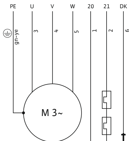
Fig. 7: Schéma de raccordement moteur 3~ : Démarrage direct, sonde bimétallique
