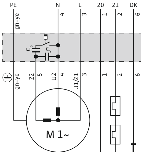
Fig. 6: Schéma de raccordement moteur 1~
