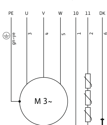
Fig. 8: Schéma de raccordement moteur 3~ : Démarrage direct, capteur PTC
