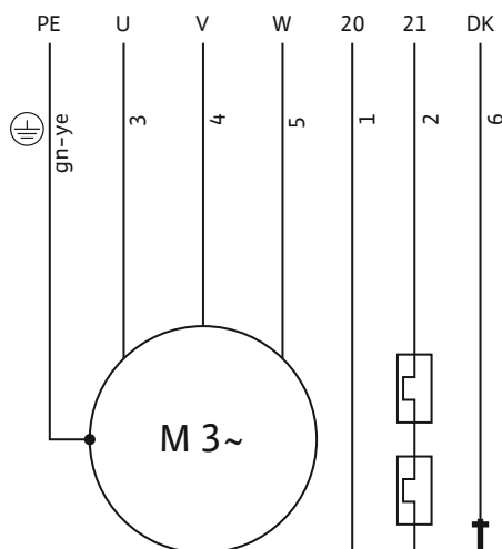
Fig. 7: Schéma zapojení 3~ motoru: Přímý start, bimetalový senzor
