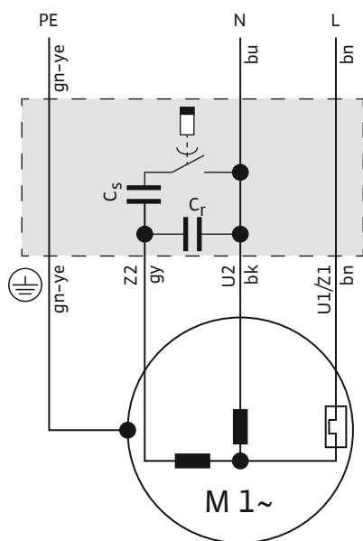
Fig. 6: Aansluitschema 1~motor
