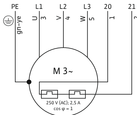
Fig. 7: Aansluitschema 3~motor
