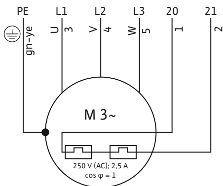
Fig. 5: Aansluitschema 3~-motor
