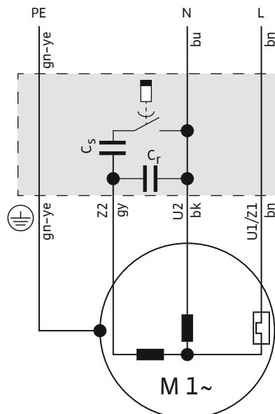
Fig. 4: Aansluitschema 1~-motor
