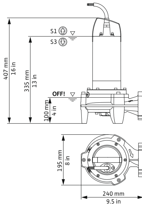
Fig. 3: Inbouwmaten
