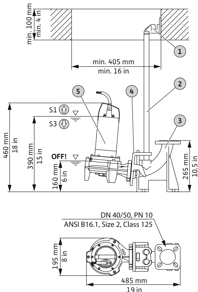
Fig. 2: Overzicht van de onderdelen en inbouwmaten
