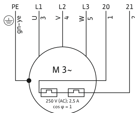
Fig. 7: Schemat połączeń silnika 3~
