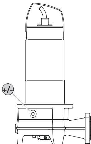
Fig. 8: Komora uszczelnienia: Wymiana oleju
