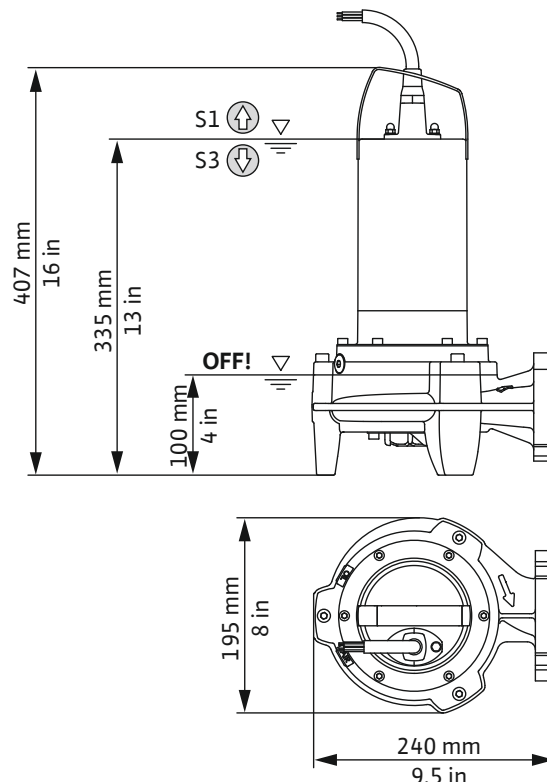
Fig. 3: Dimensions de montage
