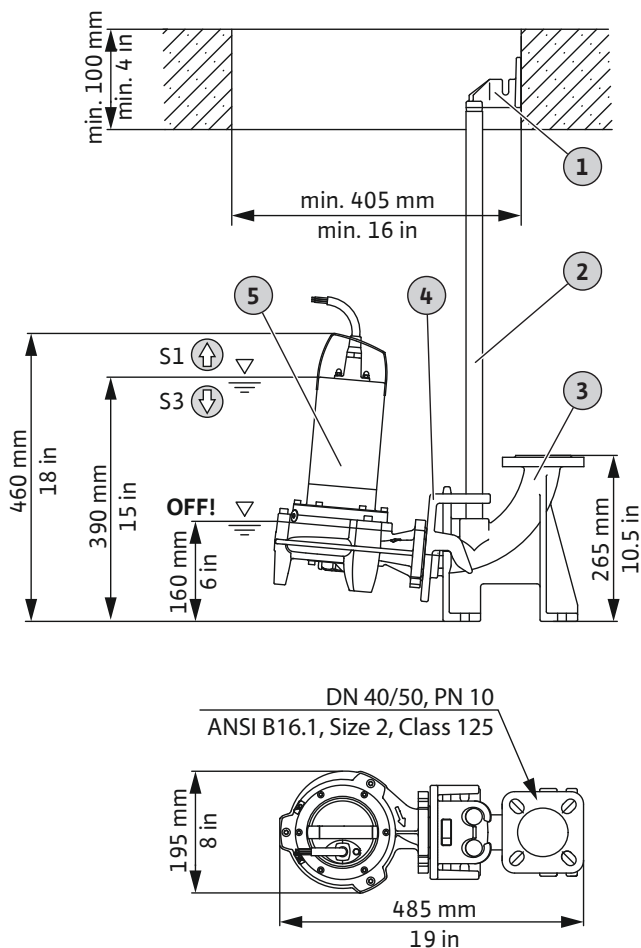
Fig. 2: Aperçu des composants et dimensions de montage
