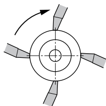
Fig. 15: Verifica dell'allineamento assiale con un calibro a corsoio - controllo perimetrale
