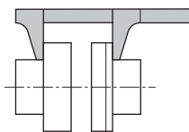
Fig. 14: Verifica dell'allineamento assiale con un calibro a corsoio
