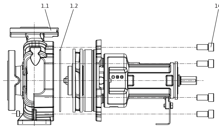
Fig. 27: Inserire l'unità ad innesto
