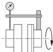
Fig. 12: Verifica dell'allineamento radiale con un comparatore
