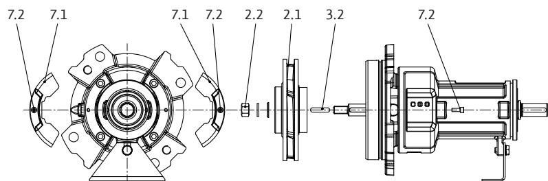
Fig. 17: Smontaggio dell'unità ad innesto
