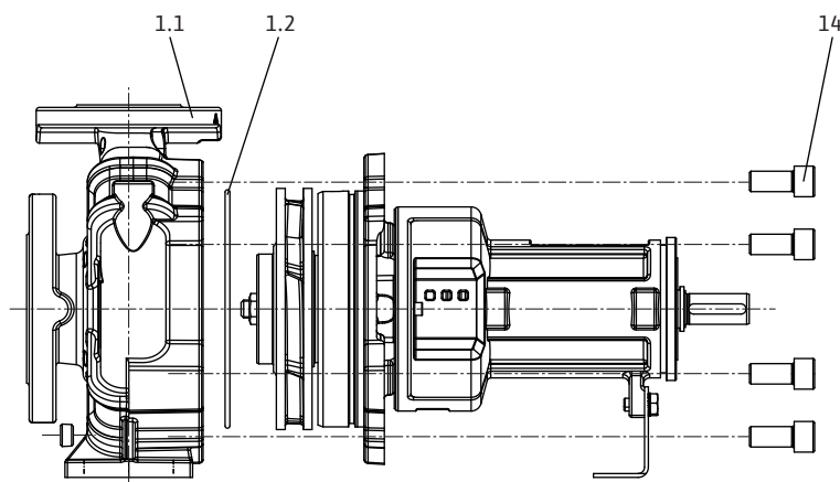
Fig. 16: Estrazione dell'unità ad innesto
