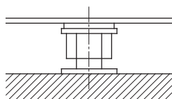
Fig. 8: Viti di livellamento sulla superficie del basamento
