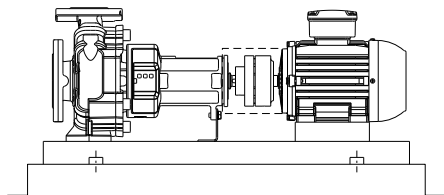
Fig. 6: Installazione del gruppo su basamento in cemento
