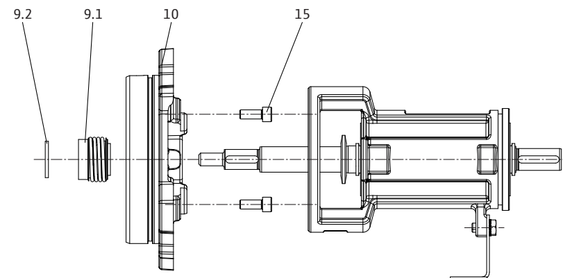
Fig. 25: Versione con tenuta meccanica
