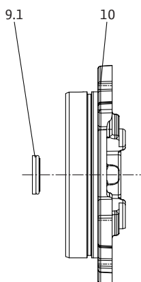
Fig. 19: Coperchio del corpo, tenuta meccanica
