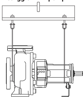
Fig. 4: Fissaggio della pompa
