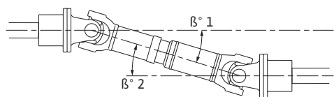
Fig. 1: Albero cardanico; assi centrali parallelamente sfalsati
