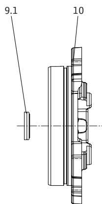
Fig. 24: Coperchio del corpo, tenuta meccanica
