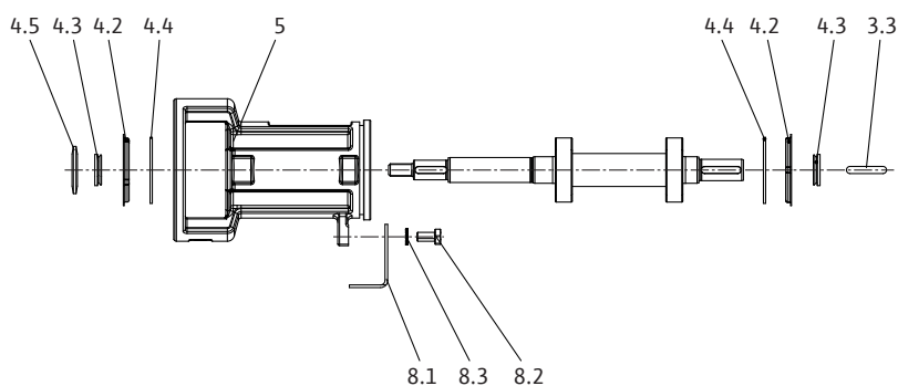
Fig. 20: Supporto cuscinetto
