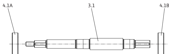
Fig. 22: Albero
