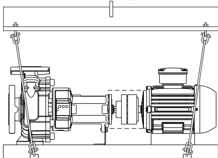
Fig. 5: Fissaggio del gruppo
