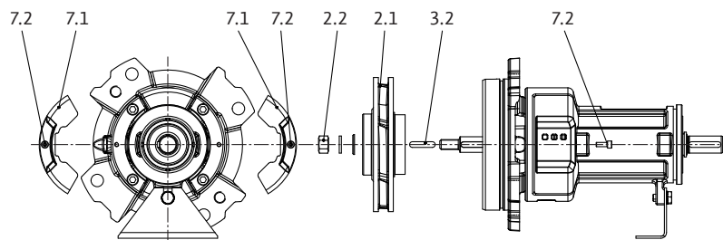
Fig. 26: Montaggio dell'unità ad innesto
