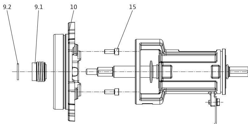
Fig. 18: Versione con tenuta meccanica
