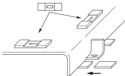
Fig. 9: Livellamento e allineamento del basamento
