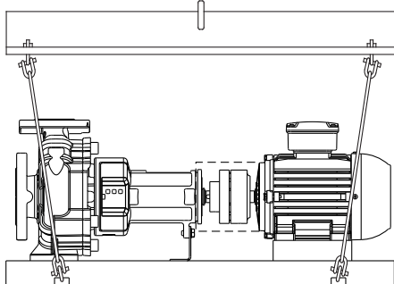
Fig. 5: Fixarea agregatului
