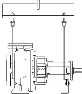
Fig. 4: Fixarea pompei
