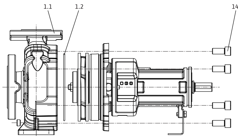
Fig. 16: Scoaterea unității de împingere
