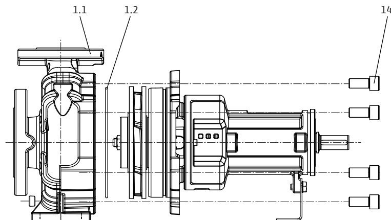
Fig. 27: Introducerea unității de împingere
