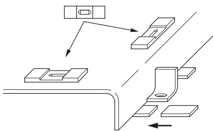
Fig. 9: Nivelarea și alinierea plăcii de bază
