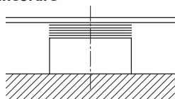
Fig. 7: Șaibe de compensare pe suprafața fundației
