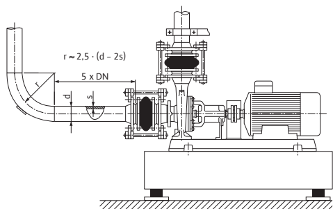
Fig. 11: Racordarea fără tensiune a pompei, tronsonul amortizor în aval și în amonte de pompă
