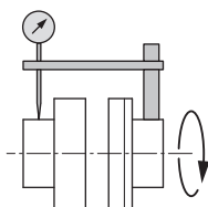
Fig. 12: Verificarea alinierii radiale cu un comparator
