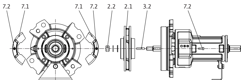
Fig. 17: Demontarea unității de împingere
