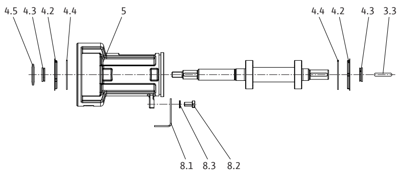
Fig. 20: Suport lagăr
