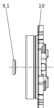
Fig. 24: Capacul carcasei, etanșarea mecanică
