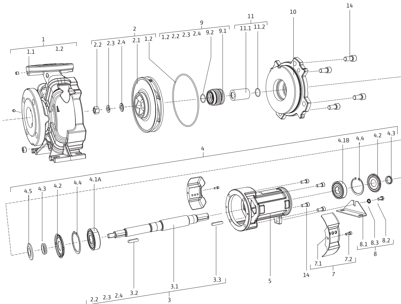
Fig. 29: Pompă cu etanșare mecanică
