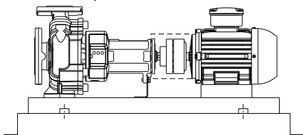
Fig. 6: Amplasarea pe fundație a agregatului
