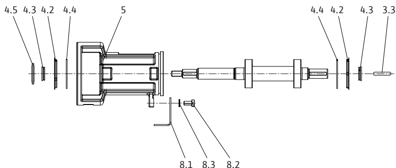
Fig. 23: Suport lagăr
