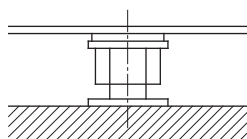
Fig. 8: Șuruburi de nivelare pe suprafața fundației
