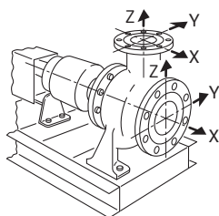
Fig. 2: Forțe și cupluri admise la nivelul flanșelor pompei – pompă din fontă cenușie
