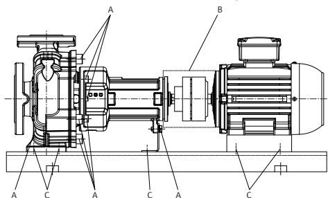
Fig. 28: Cupluri de strângere a șuruburilor
