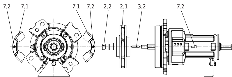
Fig. 26: Montarea unității de împingere
