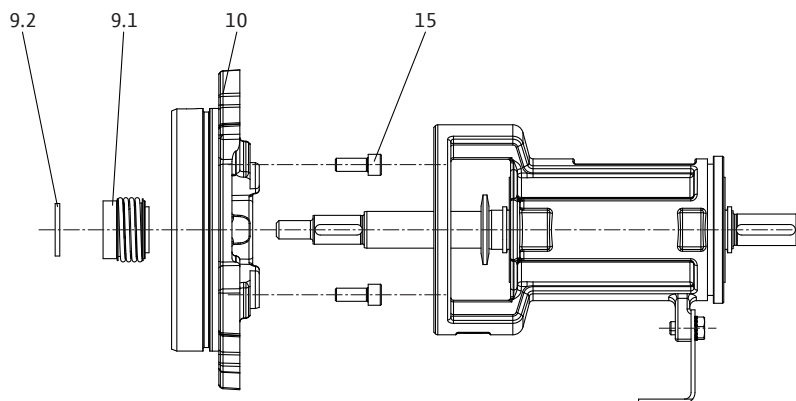
Fig. 18: Versiunea cu etanșare mecanică
