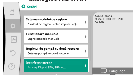
Fig. 66: Interfețe externe
