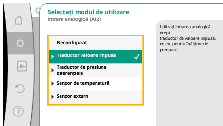
Fig. 73: Dialog de setare
