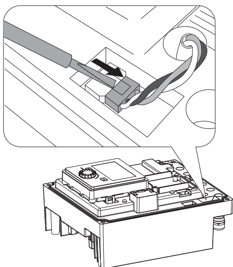
Fig. 104: Deconectarea cablului de conectare al ventilatorului modului
