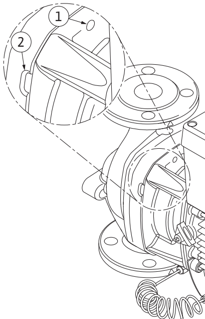
Fig. 99: Găuri filetate și fante pentru împingerea ansamblului motor cu rotor hidraulic din carcasa pompei
