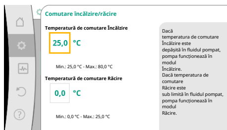
Fig. 51: Comutare încălzire/răcire_Temperaturi de comutare
