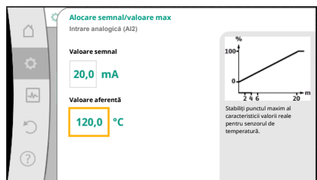
Fig. 86: Atribuire semnal max./valoare traductor de valoare reală
