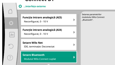
Fig. 87: Setarea interfeței Bluetooth
