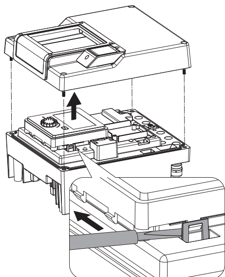
Fig. 107: Demontați capacul modulului; eliberați unitatea de display și operare din elementul de blocare
