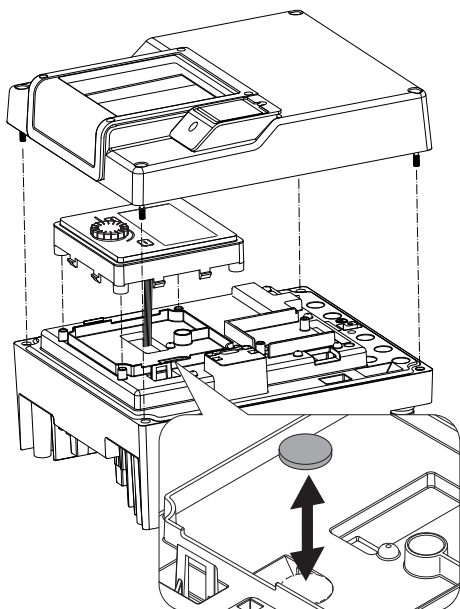
Fig. 108: Ridicarea unității de display și operare, înlocuirea bateriei
