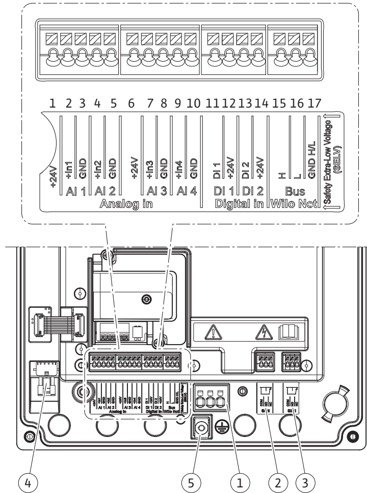
Fig. 19: Presentare generală a bornelor în modul
