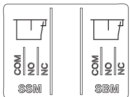
Fig. 23: Borne pentru SSM și SBM
