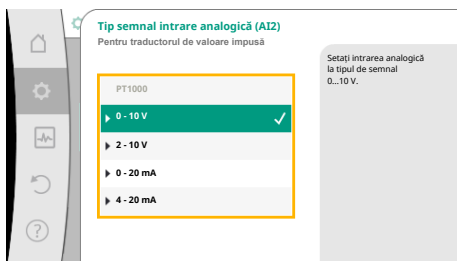
Fig. 74: Tipul semnalului
