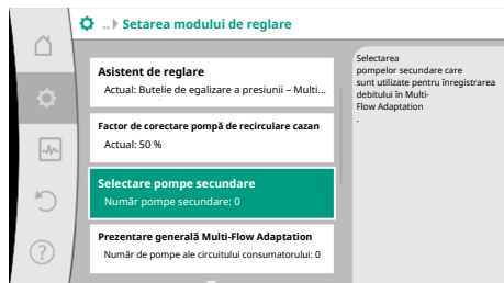
Fig. 57: Asistent de reglare – selectare pompe secundare
