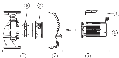
Fig. 3: Subansambluri funcționale
