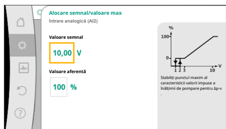
Fig. 81: Alocare semnal/valoare max
