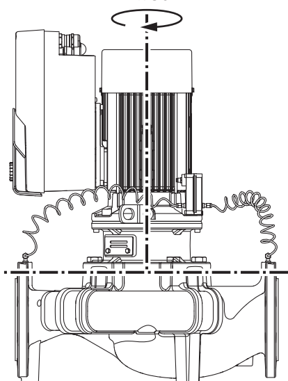
Fig. 9: Poziții de montare admise la arborele motor dispus vertical
