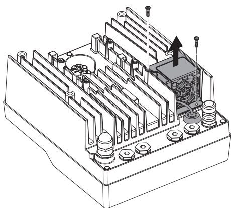
Fig. 105: Demontarea ventilatorului modului
