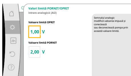
Fig. 79: Valori limită pentru comandă PORNIT/OPRIT prin semnale analogice
