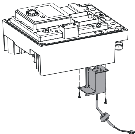
Fig. 106: Scoateți ventilatorul modulului, inclusiv cablul și garnitura din cauciuc
