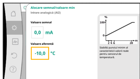
Fig. 85: Atribuire semnal min./valoare traductor de valoare reală
