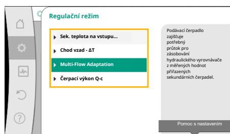
Fig. 55: Příklad Regulační režim „Multi-Flow Adaptation“
