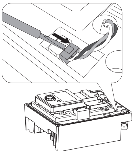
Fig. 104: Uvolnit přívodní kabel ventilátoru modulu
