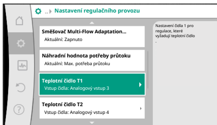
Fig. 61: Směšovač Multi-Flow Adaptation: Teplotní čidlo
