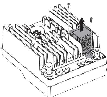
Fig. 105: Demontáž ventilátoru modulu
