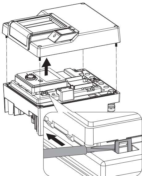
Fig. 107: Odmontování víka modulu; Uvolněte displej a řídicí jednotku ze zajišťovacího mechanismu
