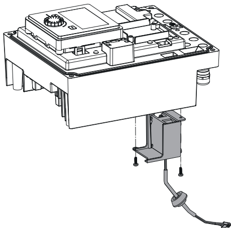
Fig. 106: Vyjměte ventilátor modulu včetně kabelu a pryžového těsnění
