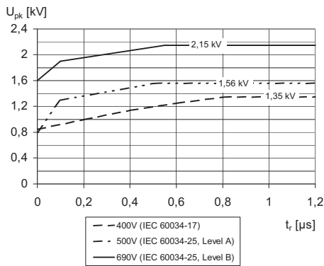
Fig. 7: Artış süresinin bir fonksiyonu olarak iki hattın klemensleri arasında izin verilen pals gerilimi U_{pk} (gerilim yansıması ve sönümlenme dahil) için sınır eğrisi t_r
