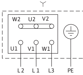
Fig. 5: Y devresi
