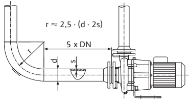
Fig. 4: Pompanın önündeki ve arkasındaki sönümlleme hattı
