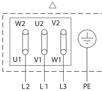
Fig. 6: Δ devresi
