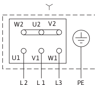
Fig. 5: Σύνδεση Υ
