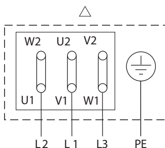
Fig. 6: Σύνδεση Δ
