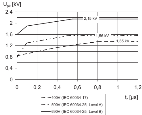
Fig. 7: Οριακή καμπύλη για την επιτρεπόμενη τάση παλμού U_{pk} (συμπεριλαμβανομένης της ανάκλασης τάσης και της απόσβεσης) μεταξύ των ακροδεκτών δύο γραμμών ως συνάρτηση του χρόνου ανόδου t_r
