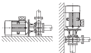
Fig. 2: Illustration af Atmos GIGA-B
