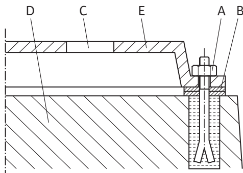
Fig. 3: Exemplo de aparafusamento da fundação
