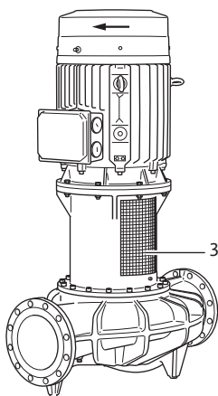
Fig. 8: Lamiera di protezione del giunto, montata
