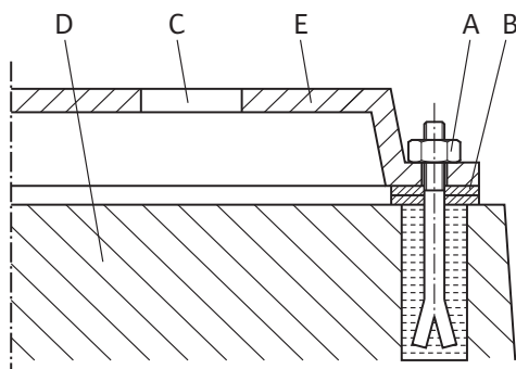
Fig. 3: Ejemplo de atornilladura a los cimientos
