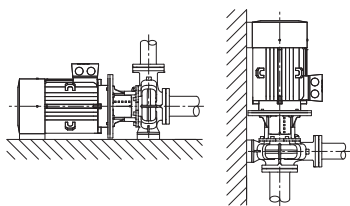
Fig. 2: Vista Wilo-Atmos GIGA-B
