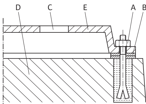
Fig. 3: Esempio di avvitamento del basamento
