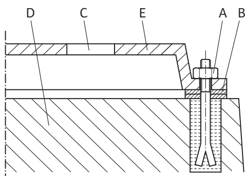
Fig. 3: Eksempel på en fundamentforskrining
