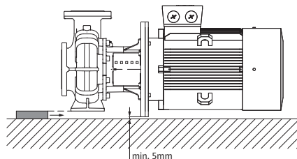
Carcasa de la bomba con apoyo
