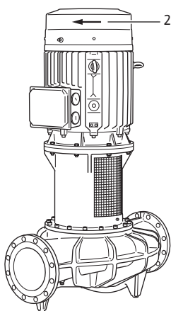
Fig. 7: Kontrol af omdrejningsretningen
