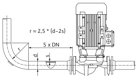
Fig. 4: Stille strækning før og efter pumpen
