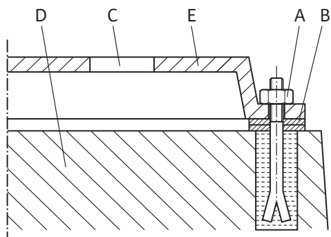
Fig. 3: Παράδειγμα για κοχλίωση θεμελίωσης
