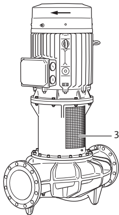
Fig. 8: Συναρμολογημένο προστατευτικό έλασμα συνδέσμου
