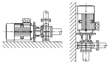
Fig. 2: Όψη Atmos GIGA-B
