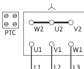
Fig. 11: Переключение Y
