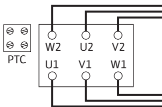
Fig. 12: Δ-схема
