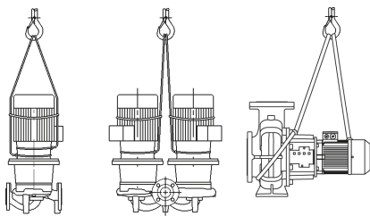
Fig. 1: Транспортировка насоса
