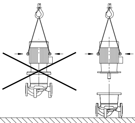
Fig. 2: Транспортировка электродвигателя
