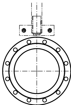
6036028 Flansch flange bride DN250 PN10 DIN2632 C / EN1092-1/11
