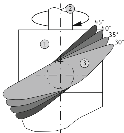
Fig. 7: Aanzethoek propellerbladen
