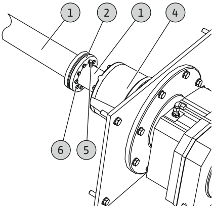
Fig. 14: Desmontaje del eje del agitador.
