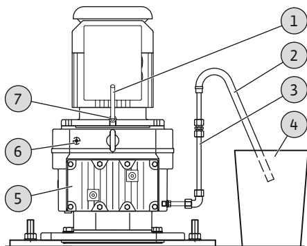
Fig. 11: Cambio de aceite
