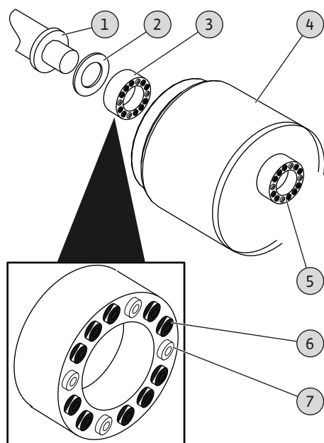
Fig. 12: Montaje/desmontaje del buje
