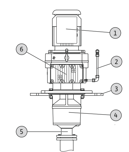
Fig. 2: Componentes de la unidad de accionamiento
