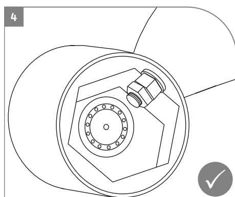
Fig. 9: Montaje de la hélice
