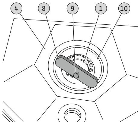
Fig. 13: Montaje del dispositivo de sujeción
