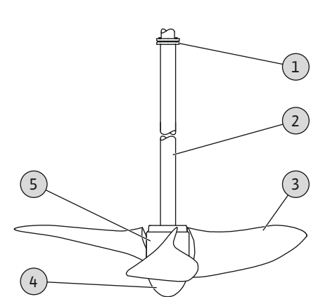
Fig. 3: Componentes del conjunto hidráulico
