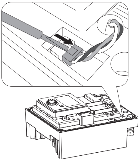
Fig. 104: Anschlusskabel des Modüllüfters lösen
