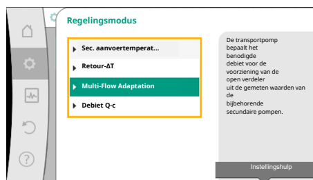
Fig. 55: Voorbeeld regelingsmodus „Multi-Flow Adaptation”
