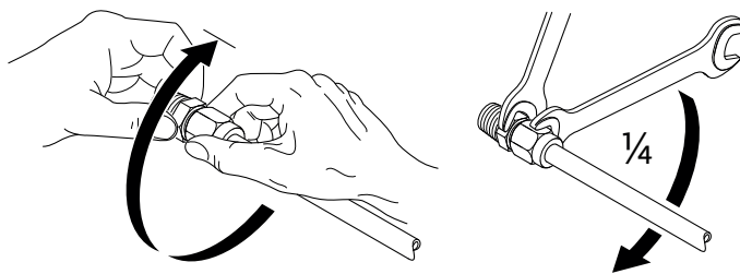
Fig. 12: Weiterdrehen der Klemmringverschraubung um 1/4 Umdrehung
