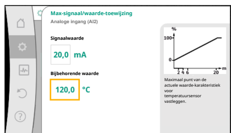
Fig. 86: Max-sigitaal/waarde-toewijzing actuele waardegever
