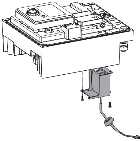
Fig. 106: Remove the module fan incl. cable and rubber sealing
