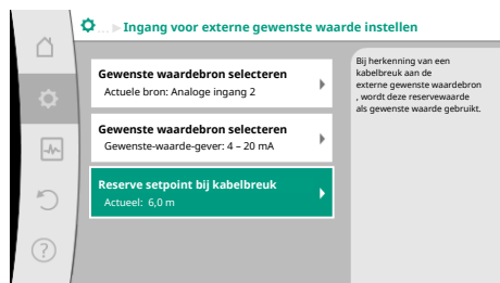
Fig. 82: Reserve setpoint bij kabelbreuk
