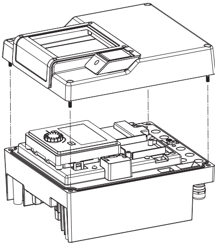
Fig. 103: Deckel des Elektronikmoduls öffnen
