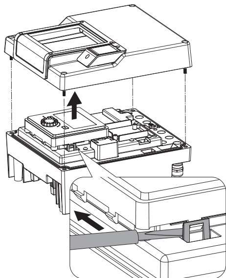
Fig. 107: Moduledeksel demonteren; display- en bedieneenheid uit de vergrendeling losmaken
