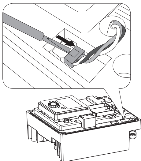
Fig. 104: Aansluitkabel van de moduleventilator losmaken
