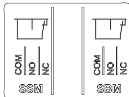
Fig. 23: Klemmen für SSM und SBM
