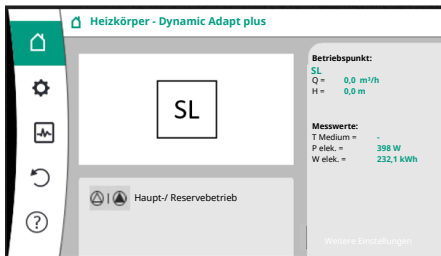
Fig. 64: Homescreen der Doppelpumpenpartner ohne montierten Differenzdrucksensor
