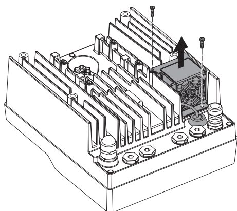
Fig. 105: Demontage van de moduleventilator
