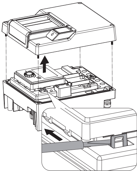
Fig. 107: Moduldeckel demontieren; Display- und Bedieneinheit aus Arretierung lösen
