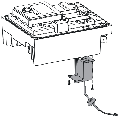
Fig. 106: Modüllüfter inkl. Kabel und Gummidichtung abnehmen
