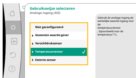
Fig. 83: Instellingsdialoog actuele waardegever
