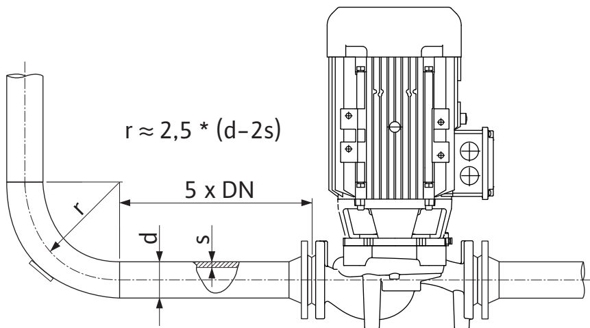
Fig. 11: Beruhigungsstrecke vor und nach der Pumpe
