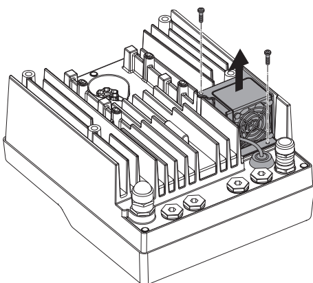
Fig. 105: Demontage des Modüllüfters
