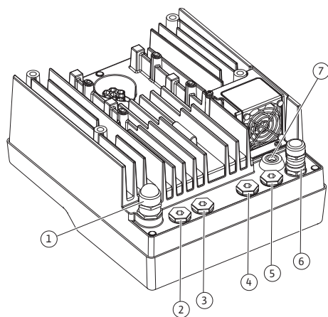
Fig. 18: Kabelverschraubungen/Kabeldurchführungen
