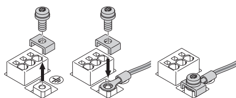
Fig. 21: Flexibele aansluitkabel
