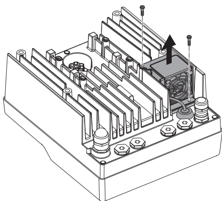
Fig. 105: Dismantling the module fan
