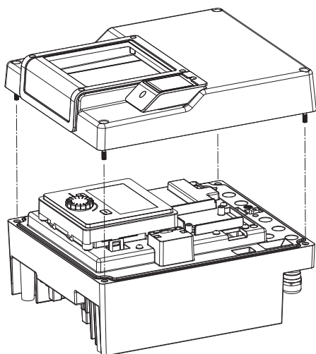
Fig. 103: Ouvrir le couvercle du module électronique
