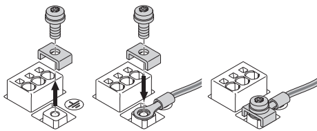
Fig. 21: Flexibles Anschlusskabel
