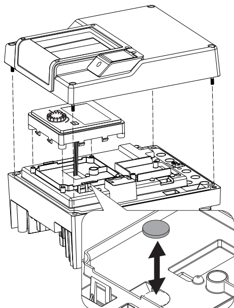
Fig. 108: Display- und Bedieneinheit anheben, Batterie austauschen
