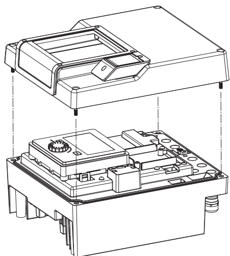
Fig. 103: Afdekking elektronica module openen
