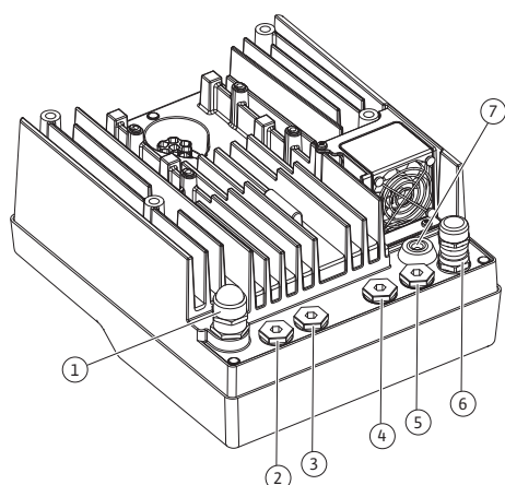
Fig. 18: Kabelschroefverbindingen/kabeldoorgangen
