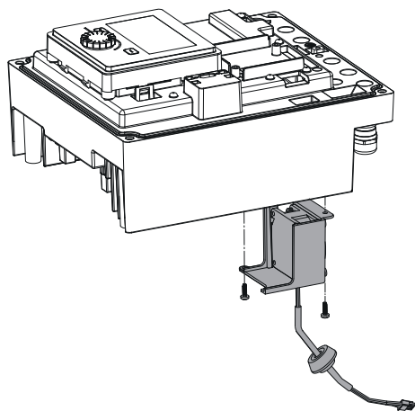
Fig. 106: Moduleventilator incl. kabel en rubberen afdichting verwijderen
