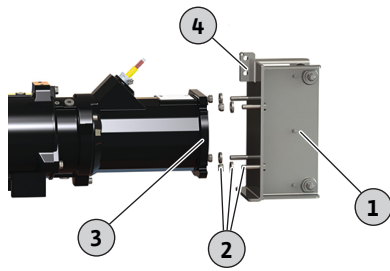
Fig. 14: Sostituire il telaio
