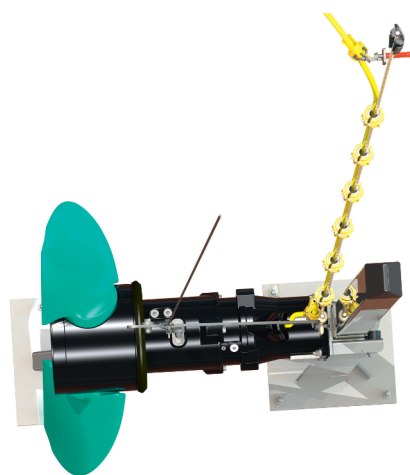
Fig. 7: Ancoraggio supplementare con fune
