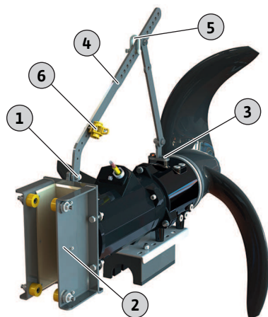
Fig. 13: Sostituire la staffa di supporto
