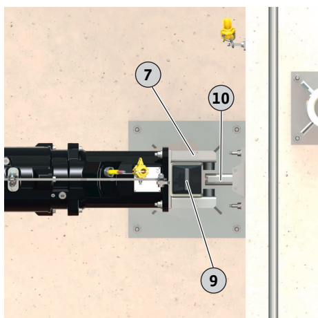
Fig. 5: Agitatore sul dispositivo di abbassamento
