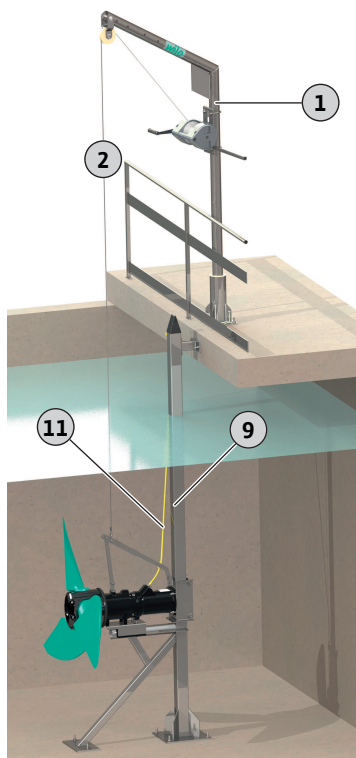
Fig. 6: Agitatore posizionato sul cavalletto
