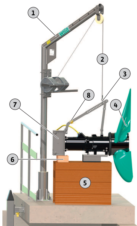
Fig. 3: Preparazione dell'agitatore
