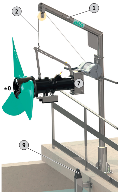
Fig. 4: Ruotare l'agitatore sopra il bacino
