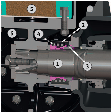
Fig. 12: Cambio della tenuta meccanica lato fluido
