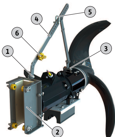
Fig. 13: Stiprinājuma loka nomainīšana
