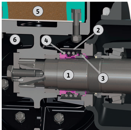
Fig. 12: Šķidrums puses gala blīvējuma nomainīšana
