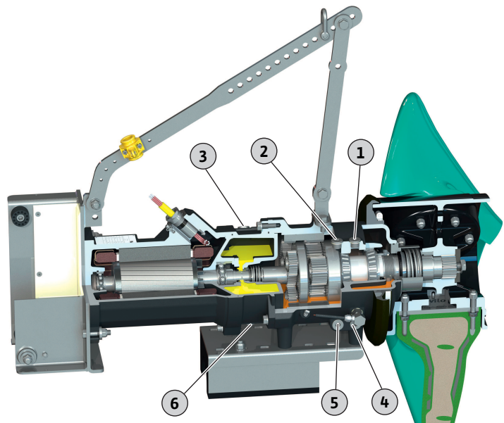
Fig. 11: Eļļas nomaiņa
