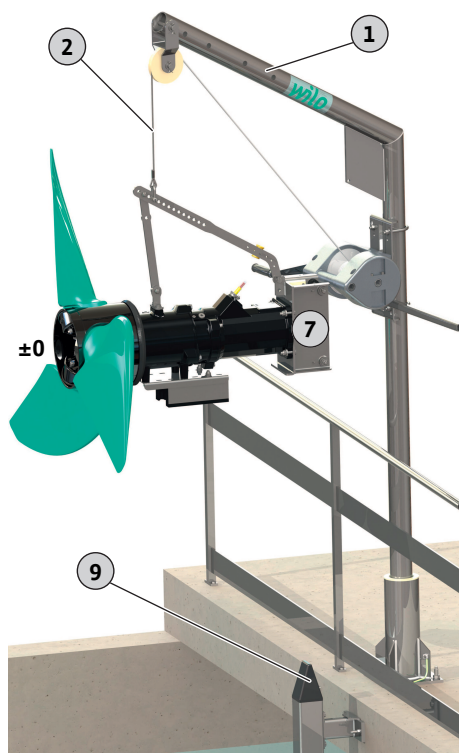
Fig. 4: Novietojiet maisītāju virs tvertnes
