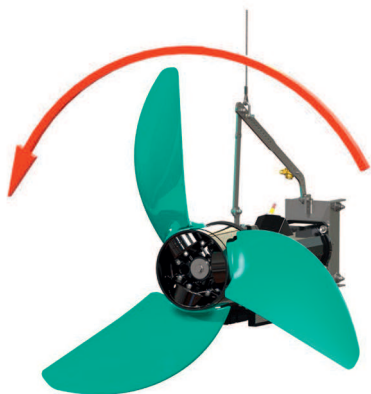
Fig. 9: Pareizs griešanās virziens TR/E 216 līdz 326-3
