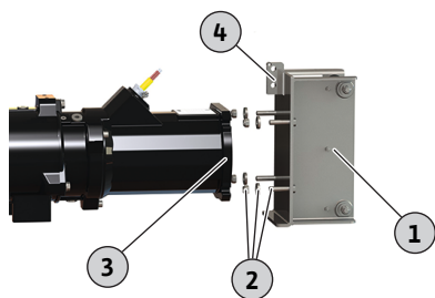
Fig. 14: Rāmja maiņa
