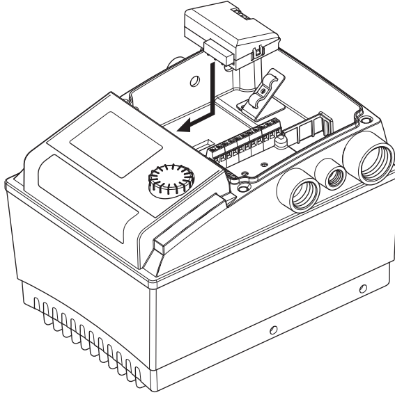
Fig. 2: Smart IF-moduulien asennus pumpuille 4 kW:iin saakka
