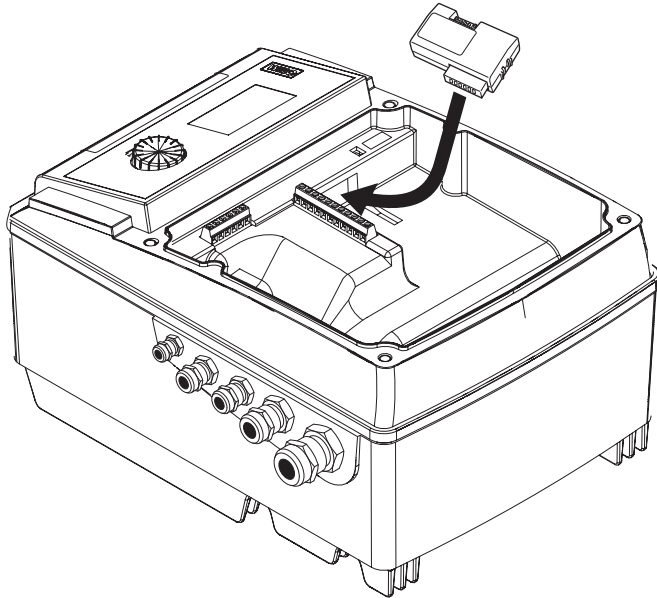
Fig. 3: Smart IF-moduulin asennus pumpuille 5–7,5 kW
