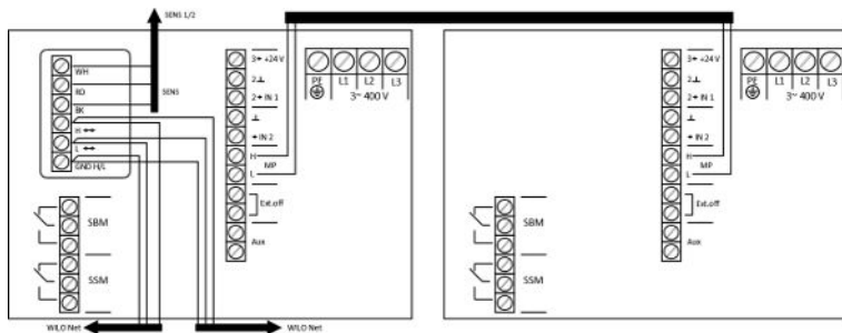
Fig. 7: Liitäntä
