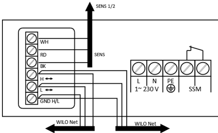
Fig. 6: Liitäntä
