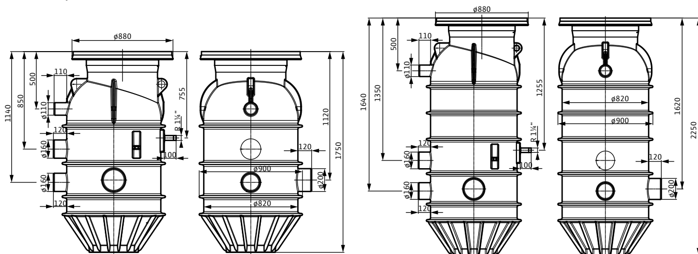
Kuva 2: Mittapiirros
