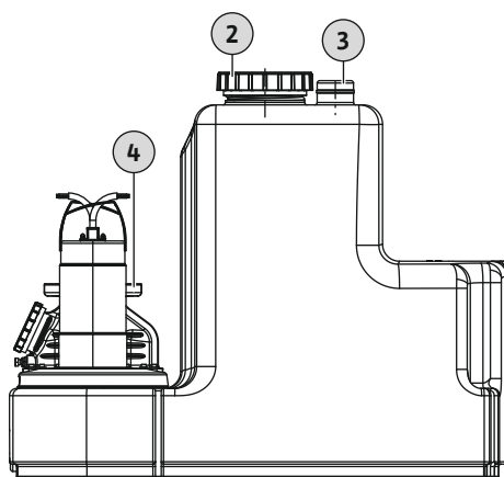
Fig. 6: Ontluchtingsaansluiting verzamelreservoir
