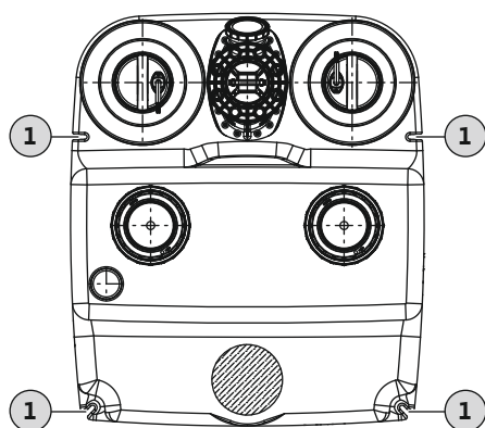
Fig. 2: Tõsteseadme pealtvaade
