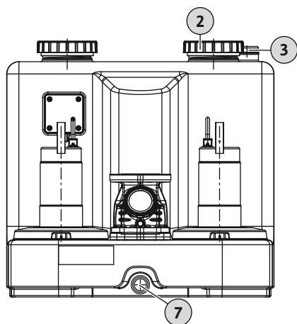
Fig. 7: Diafragmapumba lülitus
