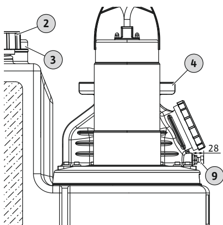
Fig. 8: Õhutuskruvi paigaldamine
