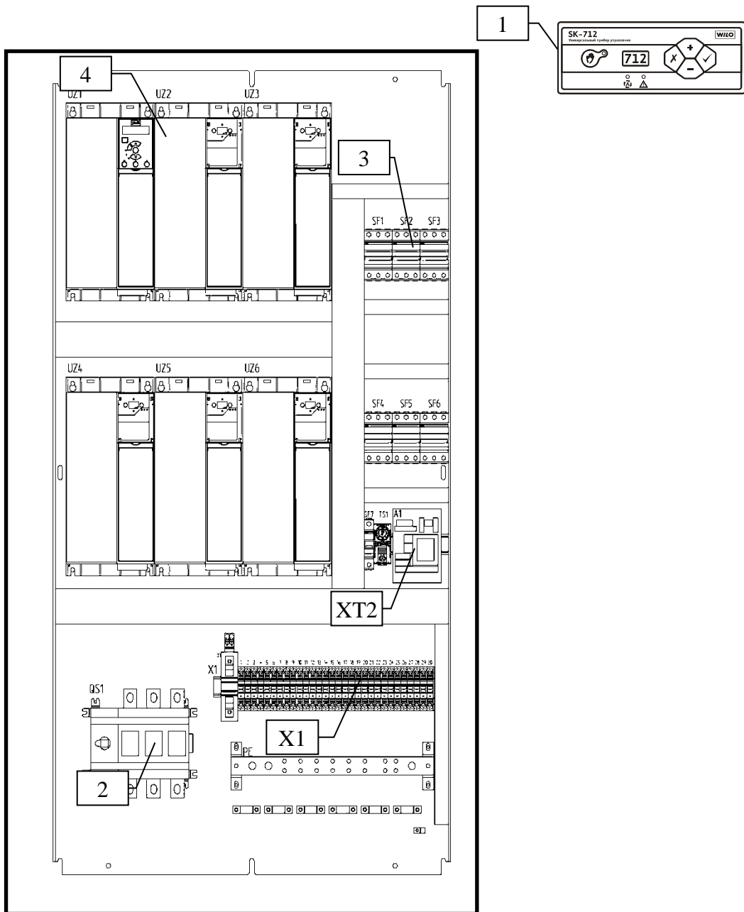
Рис. 1 Внутренний вид прибора (стандартное исполнение, без опций)
