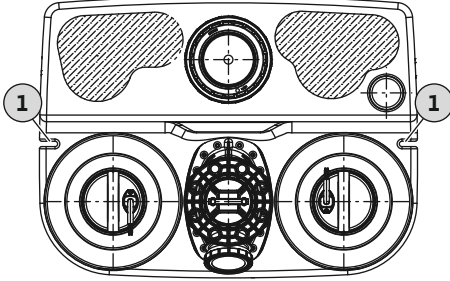
Fig. 2: Kaldırma sistemi üstten görünüm
