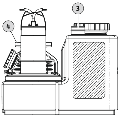
Fig. 6: Avluftsanslutning uppsamlingsbehållare
