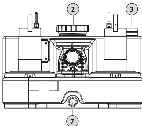
Fig. 7: Diafragminio rankinio siurblio prijungimas
