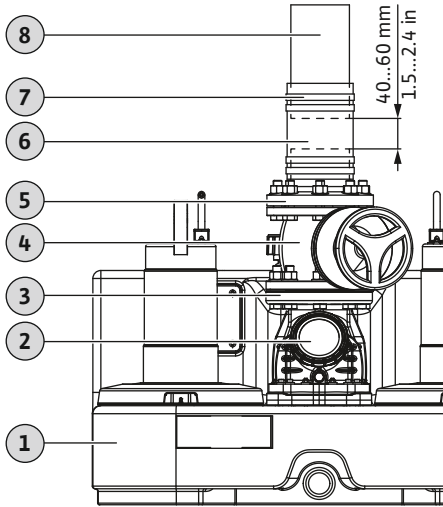
Fig. 3: Paineliitännän asennus
