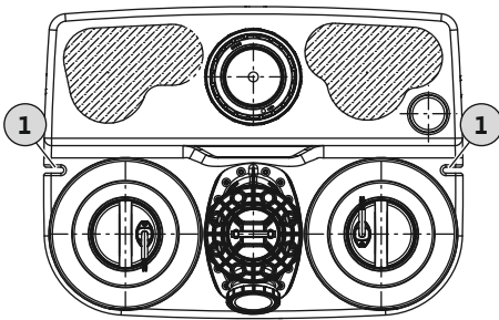
Fig. 2: Näkymä pumppaamosta ylhäältäpäin
