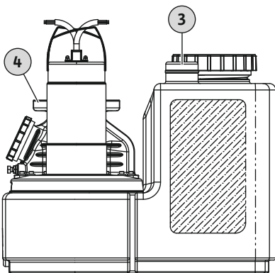
Fig. 6: Keräyssäiliön ilmanpoistoliitäntä
