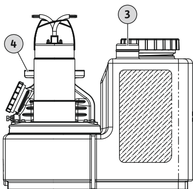
Fig. 6: Udluftningstilslutning til samlebeholder
