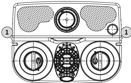
Fig. 2: Løfteanlæg set oppefra
