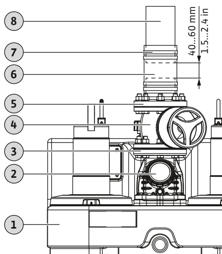
Fig. 3: Přípojka odtoku fitinku
