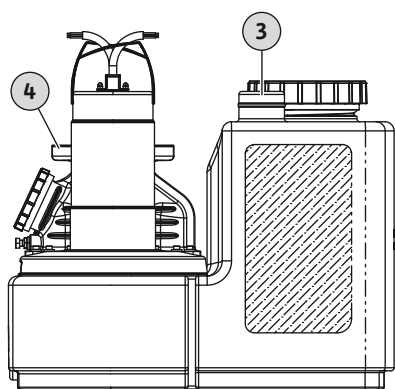
Fig. 6: Odvodňovací přípojka sběrné nádrže
